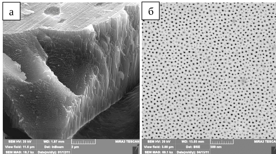
Рисунок 6.1 – Типичная микроструктура анодного оксида на сплаве А0 в стандартном серноокислом электролите (ГОСТ 9.305): а) скол оксидной пленки; б) вид сверху оксидной пленки
