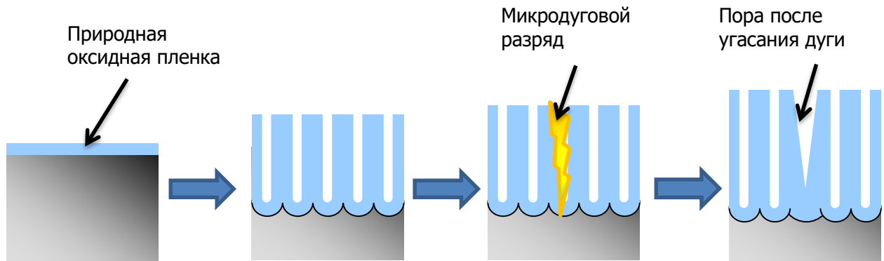
Рисунок 6.10 – Схема процесса микродугового оксидирования
