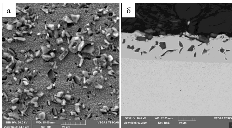
Рисунок 5.8 – Микроструктура поверхности композиционного покрытия Ni-24 об. % SiC, полученного при 2 А/дм 2 за 20 мин: а) вид сверху; б) поперечное сечение
