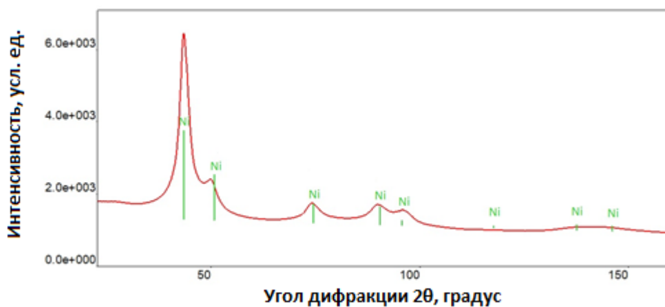
Рисунок 3.27 – Анализ электронограммы покрытия Ni-44 мас. % W, термообработанного при 500°С в течение 5 ч
