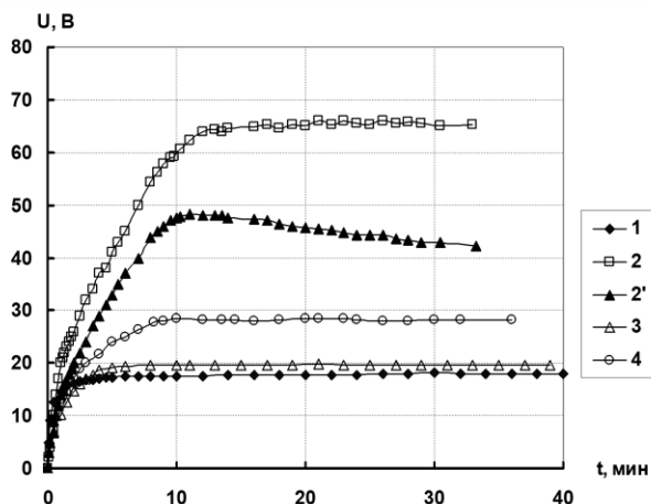
Рисунок 6.3 – Изменение напряжения на ванне при анодировании силумина АК7ч в различных электролитах при плотности тока 1 А/дм 2 . Обозначение кривых соответствуют номеру электролита в таблице 6.2 Кривые 1–4 – перемешиваемые электролиты, кривая 2' – неперемешиваемый электролит 2
