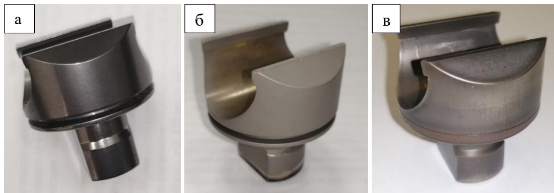
Рисунок 7.7 – Поршень гидромотора NMSE05: а) без покрытия; б) с покрытием Ni-SiC; в) после испытаний в течение 1000 ч
