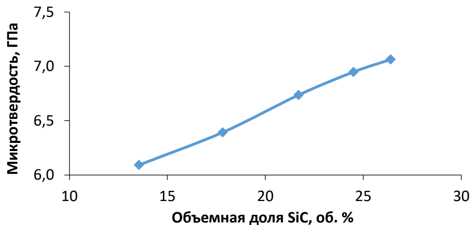
Рисунок 5.13 – Влияние содержания SiC фракции M5 в покрытии на микротвердость
