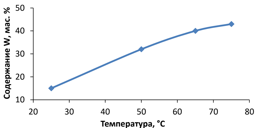
Рисунок 3.10 – Влияние температуры на состав покрытия Ni-W при осаждении из электролита 0,15 М NiSO 4 , 0,80М Na 3 Cit, 0,35М Na 2 WO 4 , 0,25 М (NH 4 ) 2 SO 4 , рН 8,0, плотность тока 5 А/дм 2
