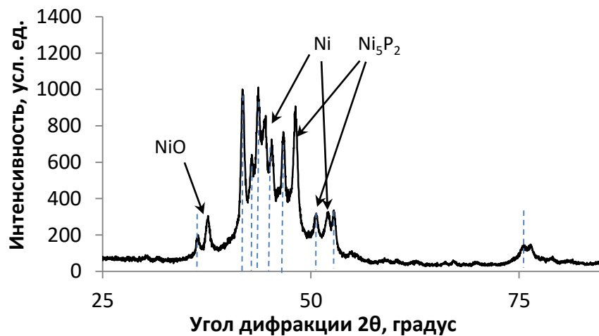
Рисунок 4.16 – Рентгеновская дифрактограмма покрытия Ni-P-W после термообработки в течение 1 ч при температуре 350 °С. Штриховыми линиями отмечено положение рефлексов фазы \text{Ni}_3\text{P}
