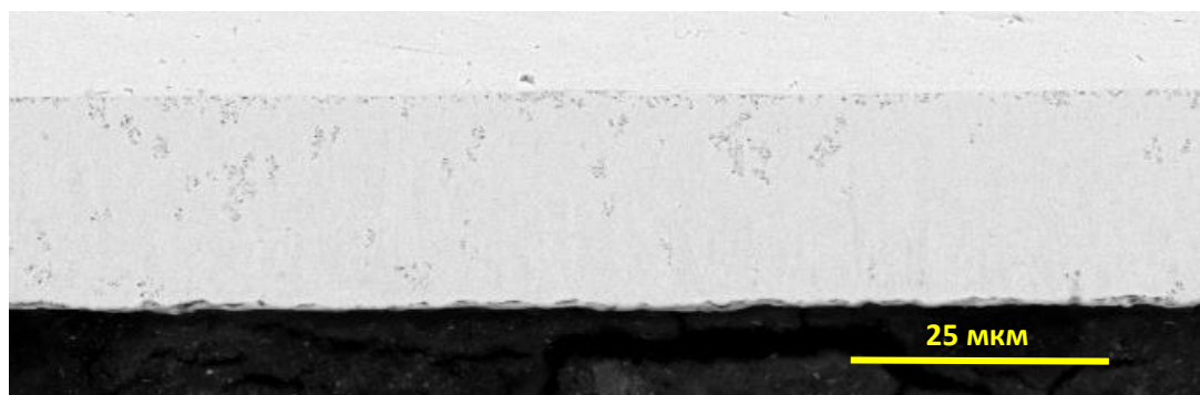
Рисунок 5.38 – Поперечное сечение КЭП никель-алмаз, осажденного концентрацией с субмикронного алмазного порошка 5 г/л
