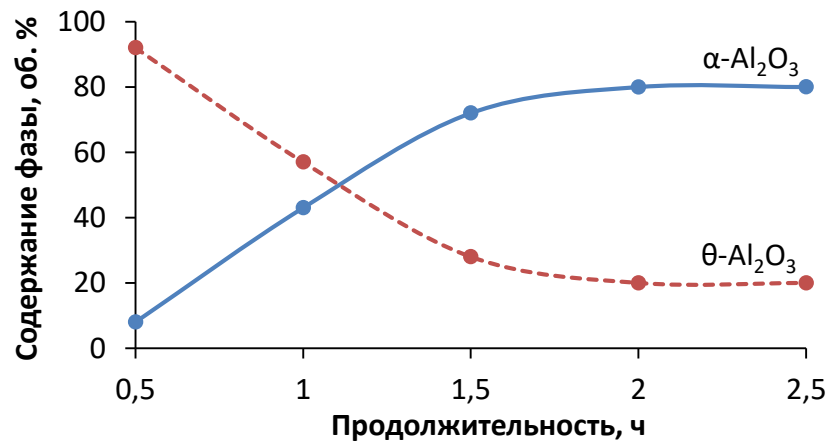
Рисунок 6.11 – Влияние продолжительности МДО в боратном электролите на фазовый состав покрытия. Плотность тока 5 А/дм 2
