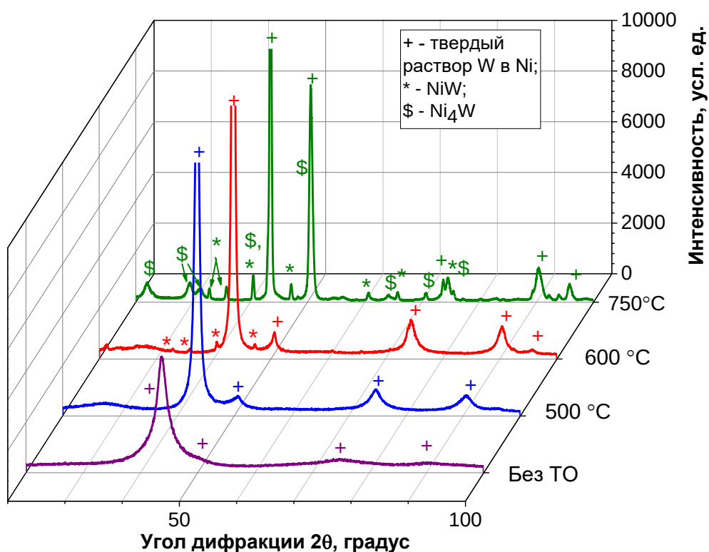
Рисунок 3.25 – Рентгеновские дифрактограммы покрытия Ni-44 мас. % W до (обозначено «без ТО») и после термообработки в течение 5 ч при различных температурах
