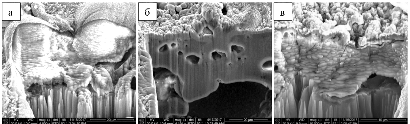
Рисунок 6.15 – Микроструктура пор МДО-покрытий, полученных в различных электролитах: а) боратный; б) силикатно-щелочной; в) силикатно-фосфатно-щелочной
