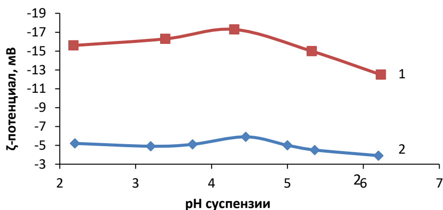
Рисунок 5.31 – Влияние pH суспензии на \zeta -потенциал алмазных частиц в среде различного состава: 1 – \text{NiSO}_4 \cdot 7\text{H}_2\text{O} 5 г/л + \text{H}_3\text{BO}_3 0,6 г/л; 2 – \text{NiSO}_4 \cdot 7\text{H}_2\text{O} 125 г/л + \text{H}_3\text{BO}_3 15 г/л
