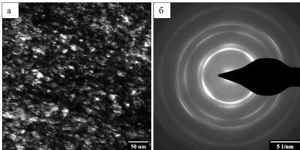
Рисунок 3.26 – Микроструктура покрытия Ni-44 мас. % W, термообработанного при 500°С в течение 5 ч: а) темнопольное изображение в рефлексе (1 1 1) Ni ; б) электронограмма
