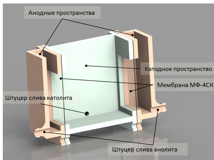
Рисунок 2.1 – Схема лабораторной мембранной ячейки для нанесения покрытий
