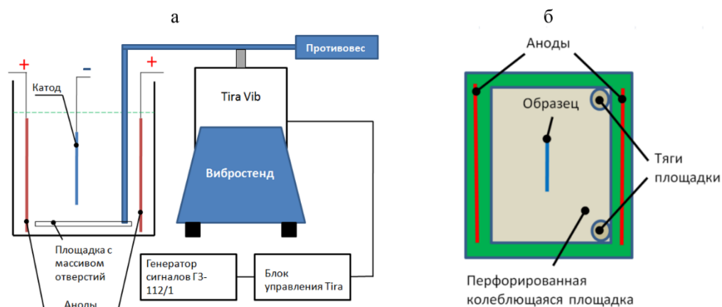
Рисунок 2.2 – Схемы установки для получения образцов композиционных покрытий (а) и расположения образца в ванне (б).
