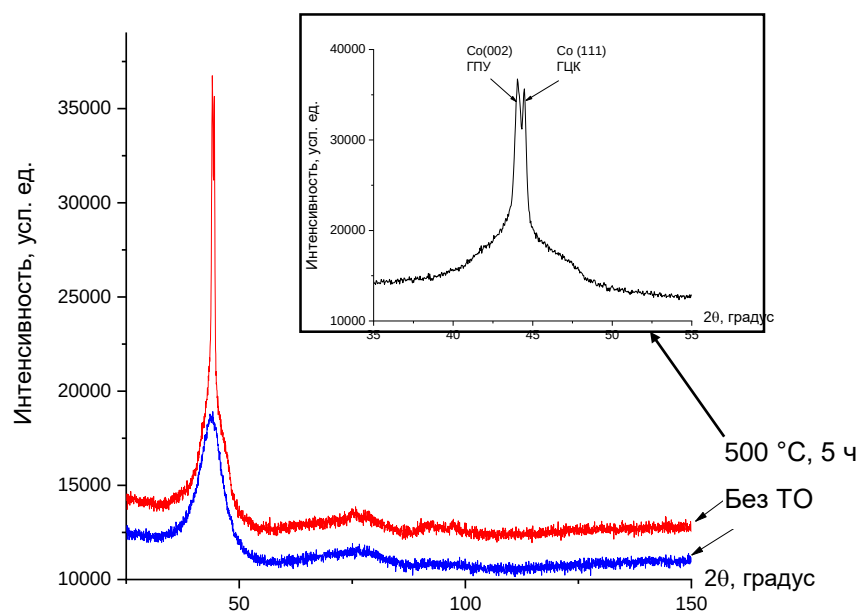
Рисунок 3.47 – Рентгеновские дифрактограммы покрытия Co-45 мас. % W, до и после термообработки при 500 °С. На врезке увеличенный участок дифрактограммы термообработанного образца
