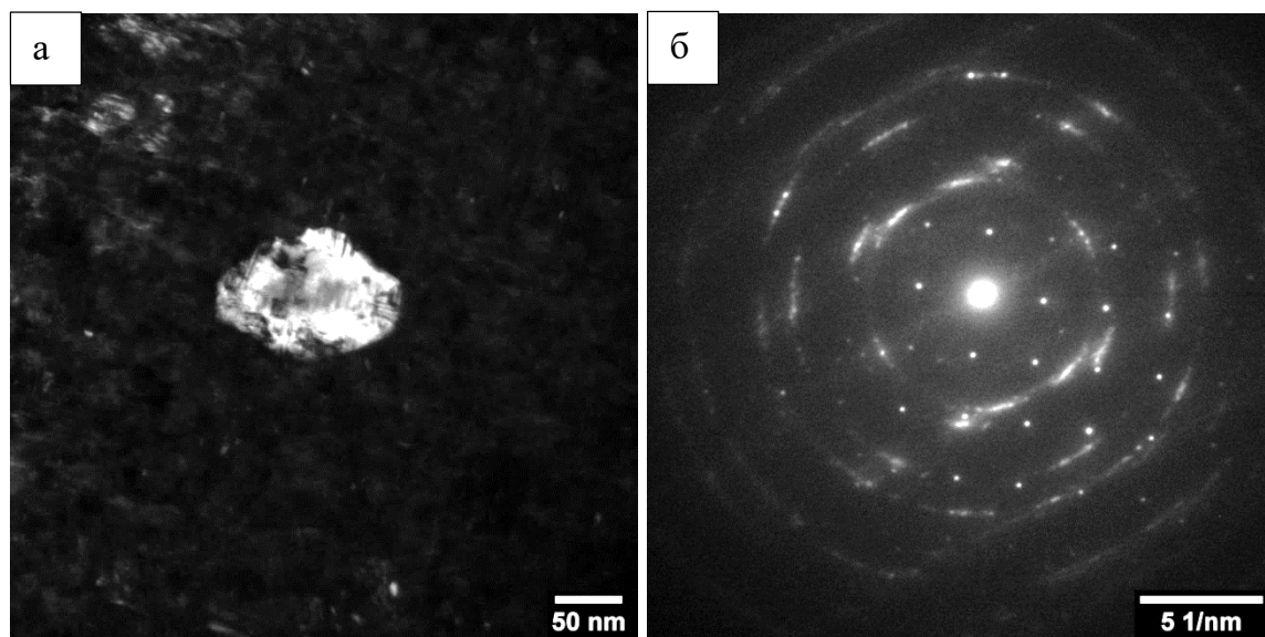
Рисунок 3.29 – Частица интерметаллида NiW в матрице из дисперсных кристаллов твердого раствора вольфрама в никеле: а) темнопольное изображение; б) электронограмма от частицы
