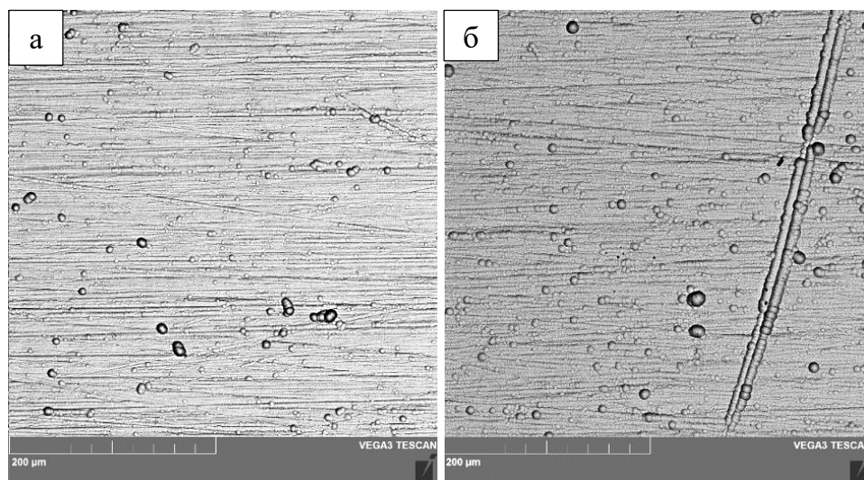
Рисунок 4.7 – Микротруктура поверхности покрытия, осажденного из цитратного электролита с 0,20 моль/л (а) и 0,10 моль/л (б) \text{NaH}_2\text{PO}_2 при плотности тока 3 А/дм 2 . Содержание фосфора 11,7 и 10,4 % соответственно
