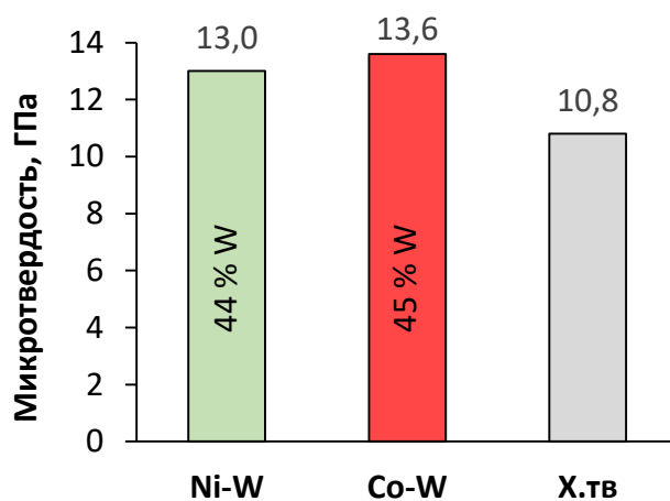
Рисунок 3.55 – Микротвердость композиционных покрытий Ni-W, Co-W, полученных термообработкой прекурсорных слоев (температура отжига 600 °С) в сравнении с твердым хромовым покрытием (максимальное значение по ГОСТ 9.303)
