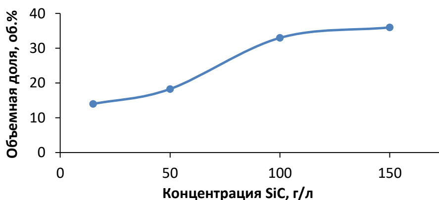
Рисунок 5.19 – Влияние концентрации частиц субмикронного порошка SiC в электролите на его объемную долю в покрытии
