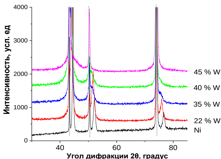
Рисунок 3.11 – Рентгеновские дифрактограммы покрытий Ni-W с различным содержанием вольфрама (в мас. %). Пунктиром обозначено положение рефлексов медной основы
