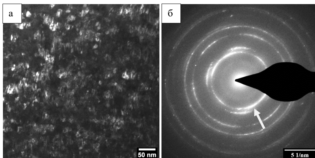
Рисунок 3.28 – Структура покрытия Ni – 44 % W, термообработанного при 600 °С в течение 5 ч: а) темнопольное изображение в рефлексе (1\ 1\ 1)_{\text{Ni}} ; б) электронограмма от места наблюдения
