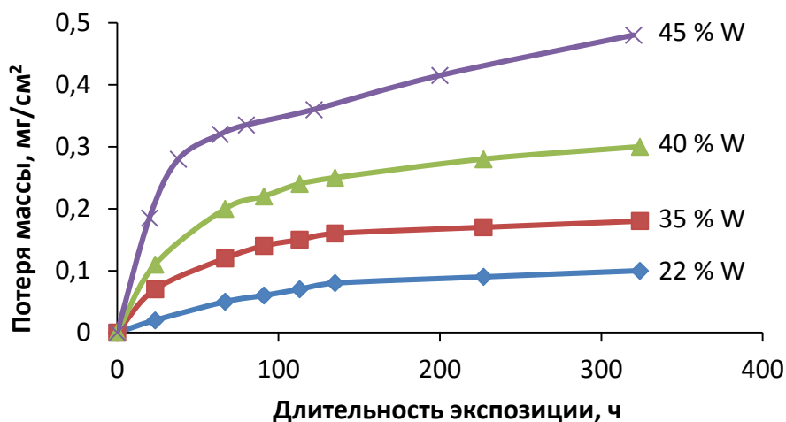
Рисунок 3.14 – Потеря массы образцов покрытий Ni-W с различным содержанием вольфрама (в мас. %) во времени при коррозии в 3,5 %-ном растворе NaCl
