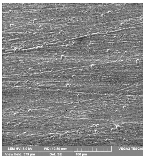
Рисунок 4.13 – Микроструктура поверхности покрытия Ni-P-W.
