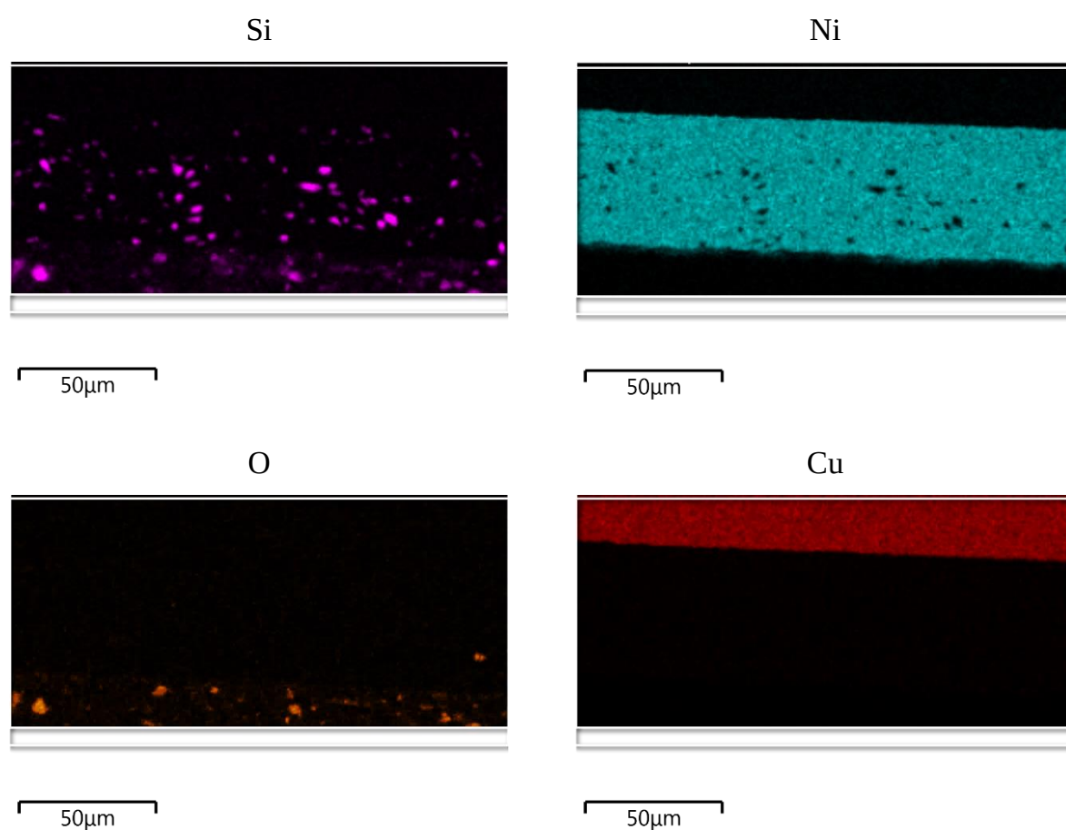
Рисунок 5.6 – Карты распределения элементов в покрытии Ni-SiC на микрошлифе
