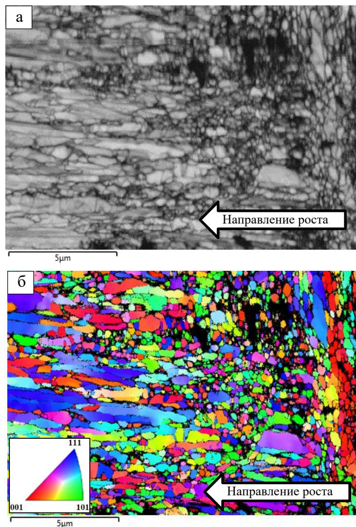
Рисунок 5.39 – Микроструктура композиционного покрытия никель-алмаз, осажденного из электролита с концентрацией субмикронного алмазного порошка 5 г/л: а) режим контраста полос Кикучи; б) карта ориентировок кристаллитов
