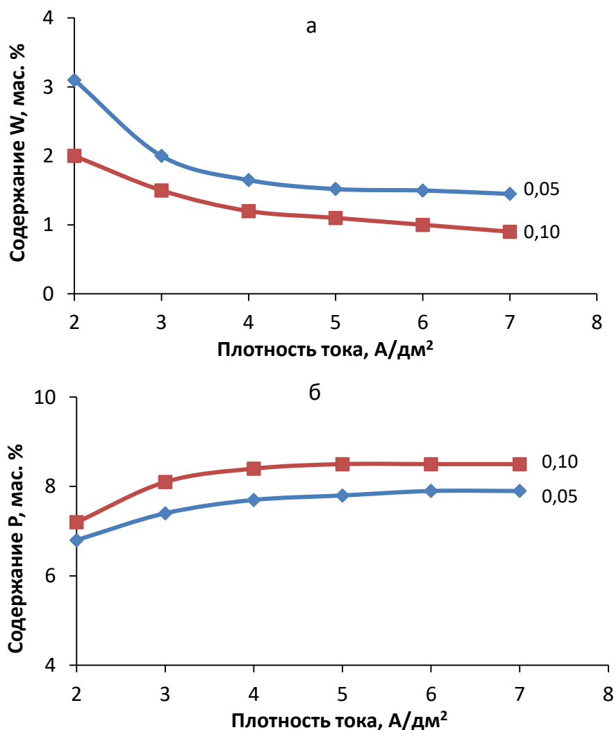
Рисунок 4.10 – Зависимость содержания вольфрама (а) и фосфора (б) в покрытии Ni-P-W от плотности тока для электролитов с различной концентрацией гипофосфита натрия, моль/л
