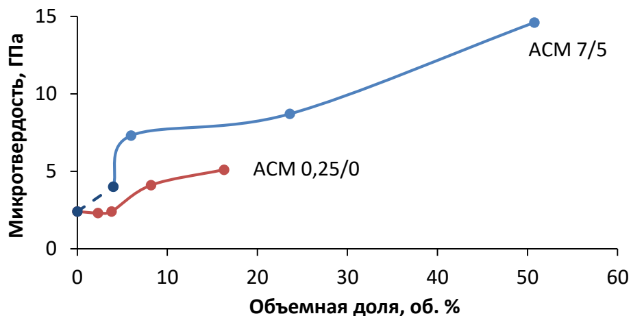
Рисунок 5.35 – Зависимость микротвердости покрытий Ni-алмаз от объемной доли армирующих частиц
