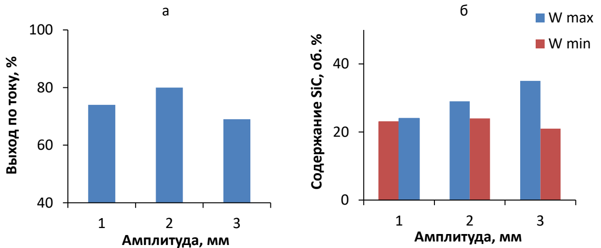
Рисунок 5.11 – Влияние амплитуды колебаний на выход по току КЭП Ni-SiC (а) и объемное содержание в нем карбида кремния (б). Частота колебаний 50 Гц
