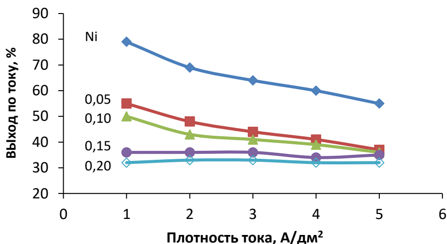
Рисунок 4.2 – Зависимость выхода по току покрытия Ni-P от плотности тока при осаждении из электролитов с различной концентрацией гипофосфита натрия, моль/л
