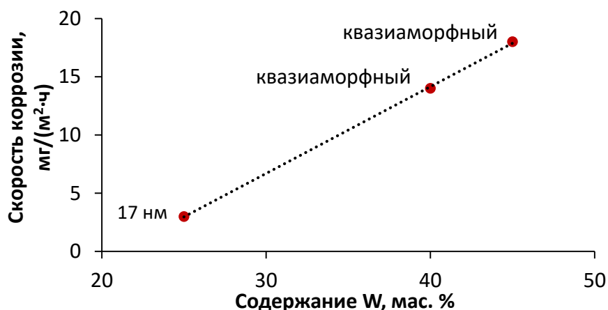
Рисунок 3.45 – Влияние содержания вольфрама на скорость коррозии электроосажденных покрытий Co-W в 3,5 %-ном растворе NaCl.
