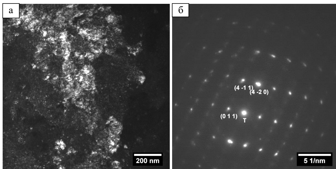
Рисунок 4.22 – Частицы \text{Ni}_3\text{P} в покрытии Ni-P-W после термической обработки на 350\text{ }^{\circ}\text{C} в течение 3 ч: а) темнопольное изображение; б) электронограмма
