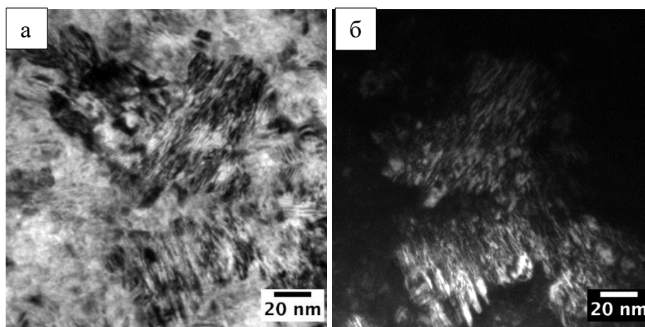
Рисунок 3.13 – Проверка результатов анализа дифрактограмм с помощью просвечивающей электронной микроскопии на образце, содержащем 22 мас. % вольфрама: а) светлопольное изображение; б) темнопольное изображение
