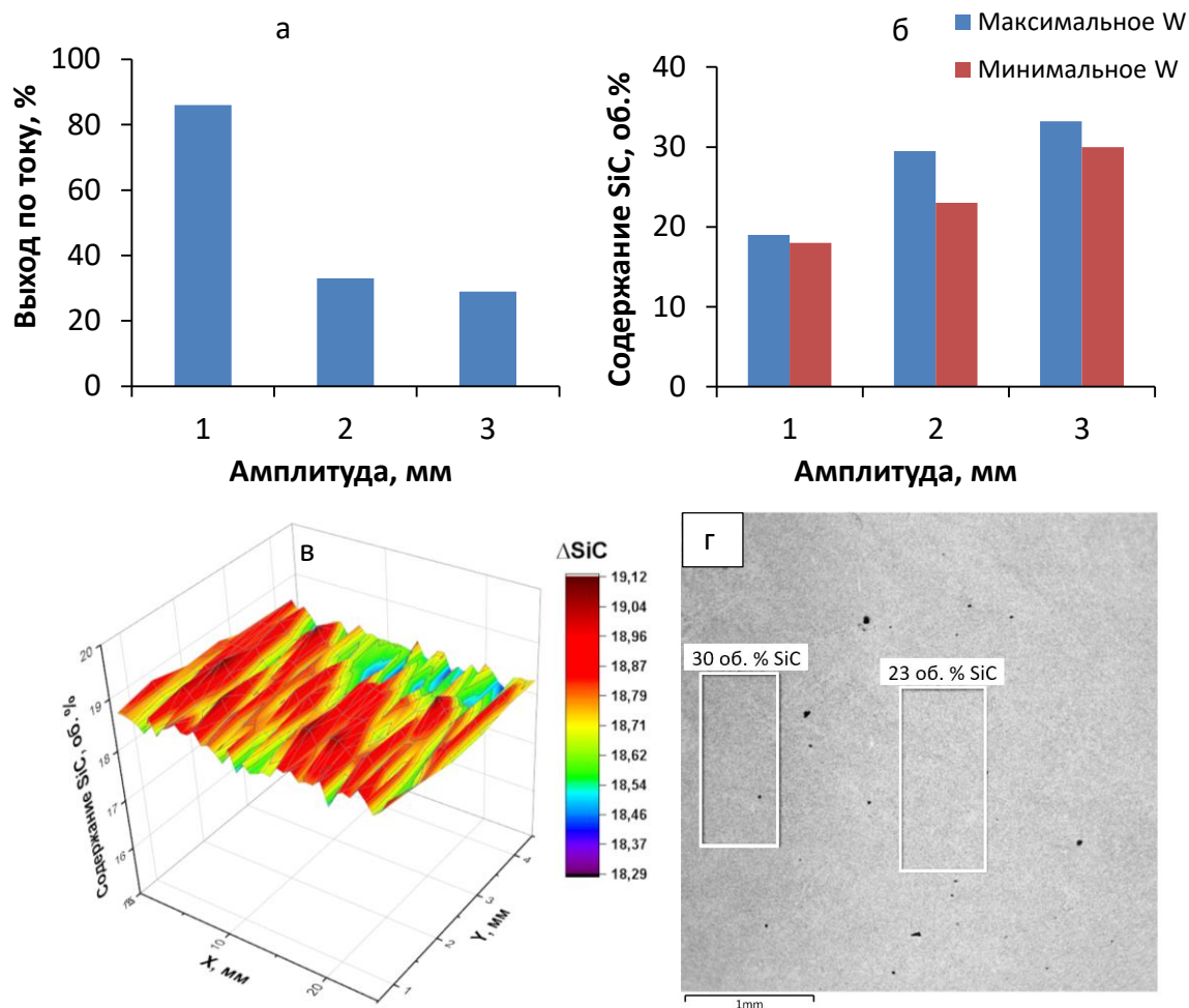
Рисунок 5.18 – Влияние амплитуды колебаний на выход по току покрытия (а), содержание карбида кремния (б) при осаждении из электролита с субмикронным порошком, карта распределения SiC по поверхности образца, полученного при амплитуде 1 мм (в) и граница между зонами с различным содержанием SiC (г) на поверхности образца, полученного при амплитуде колебаний 2 мм. Концентрация порошка 50 г/л, частота колебаний 50 Гц
