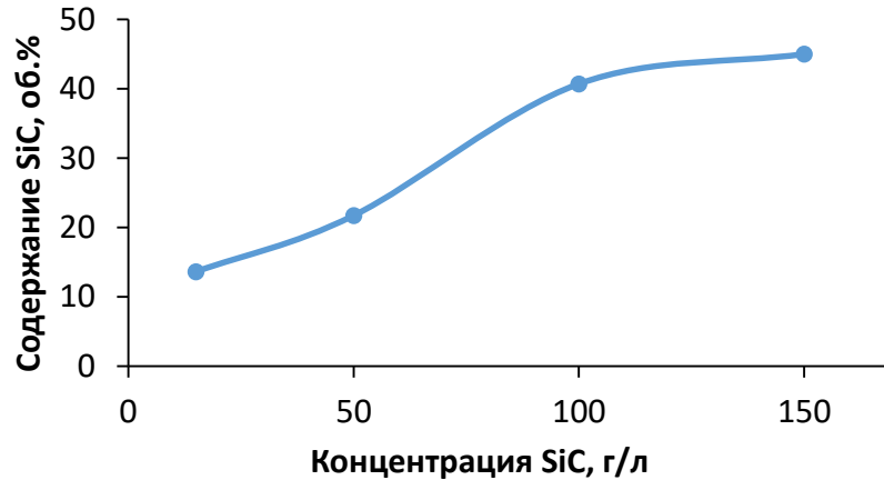
Рисунок 5.12 – Влияние концентрации порошка SiC фракции M5 в электролите на его объемную долю в покрытии
