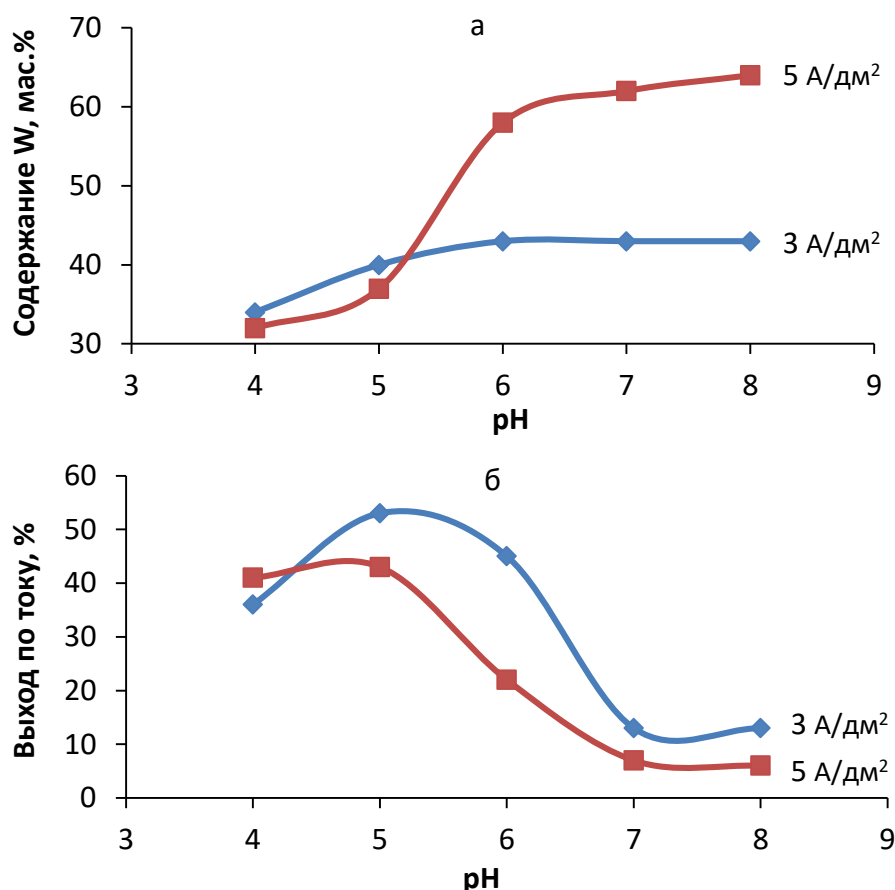
Рисунок 3.38 – Влияние рН на содержание вольфрама в покрытии Со-W (а) и выход по току (б), измеренные при осаждении покрытий при различной плотности тока
