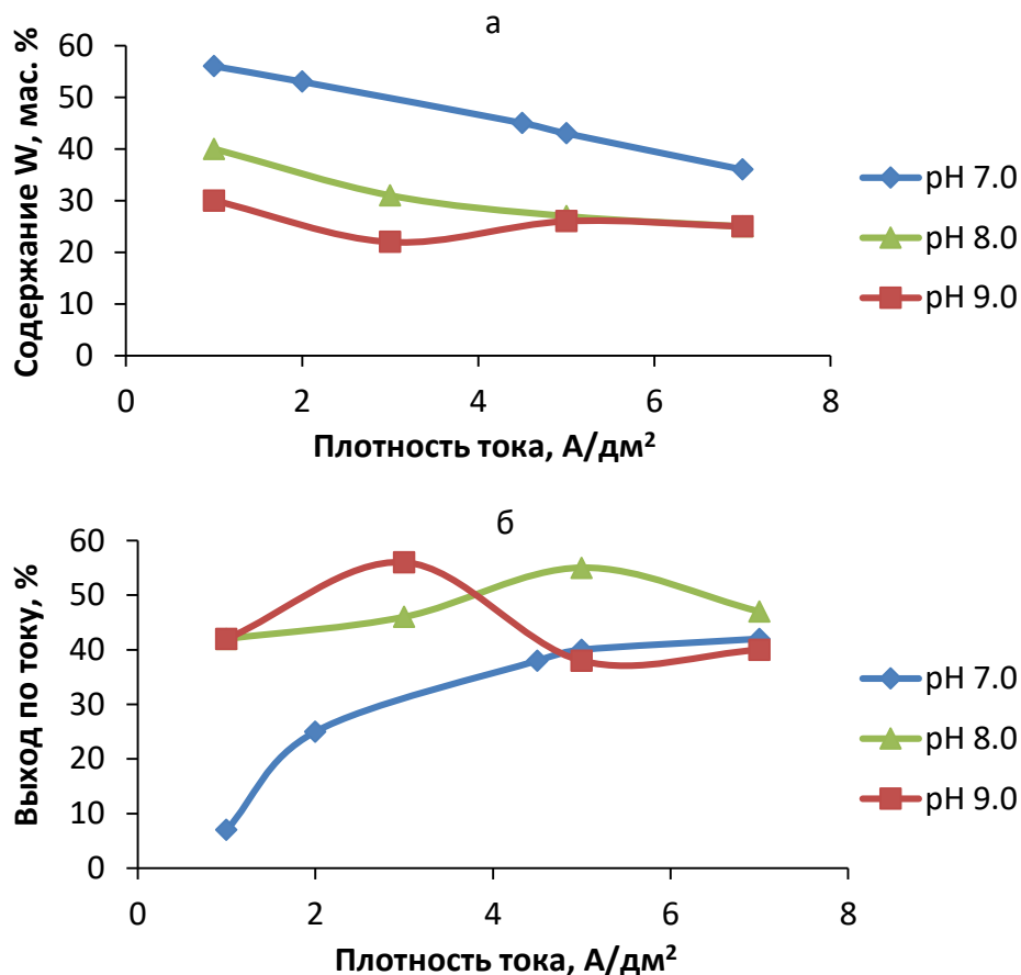
Рисунок 3.8 – Влияние величины pH на состав покрытия (а) и выход по току (б) при осаждении сплава Ni-W из электролита 0,2 М NiSO 4 , 0,8 М Na 3 Cit, 0,3 М Na 2 WO 4 , 0,25 М (NH 4 ) 2 SO 4 , температура 50 °С
