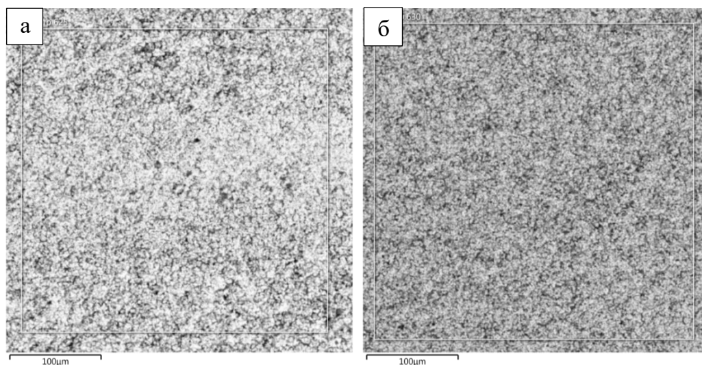
Рисунок 5.16 – Изображения поверхности образца покрытия, осажденного на медную пластину, расположенную под углом 45° ко дну ванны: а) сторона, обращенная к дну ванны; б) сторона, обращенная к зеркалу электролита
