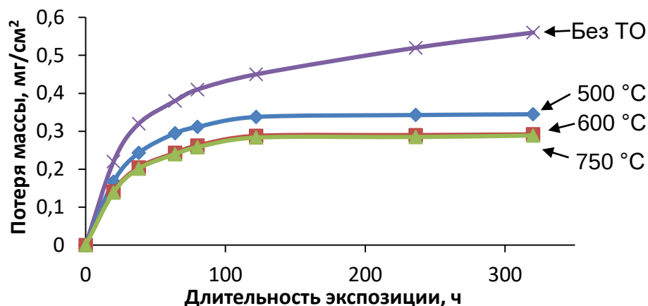
Рисунок 3.37 – Потеря массы во времени образцов с покрытием Ni-W, термообработанных при различных температурах в течение 5 ч, при коррозии в 3,5 %-ном NaCl
