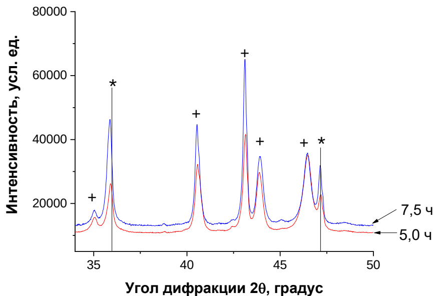
Рисунок 3.50 – Рентгеновские дифрактограммы покрытий Co-45 мас. % W, термообработанных при 750 °C
