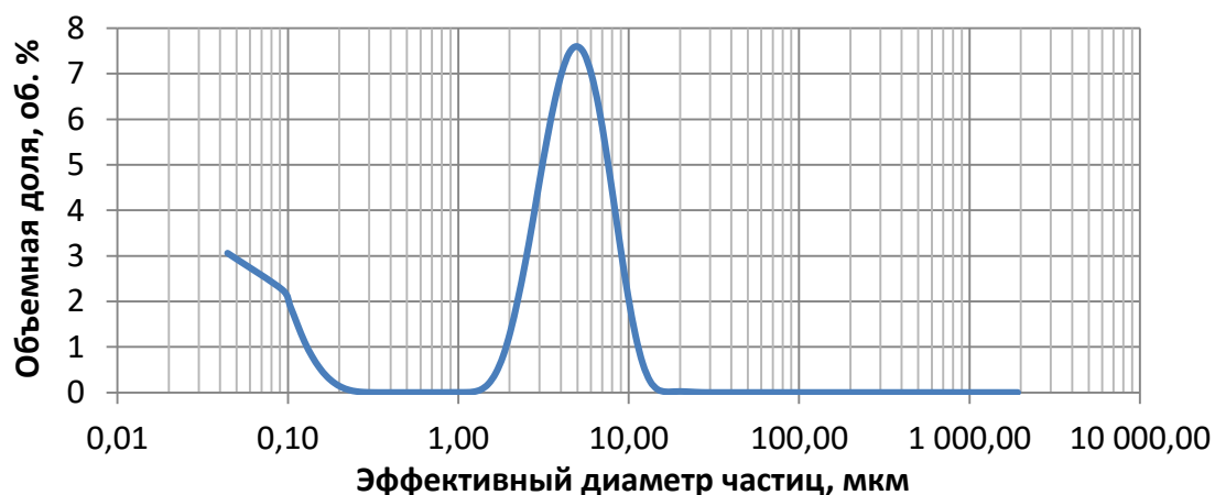
Рисунок 5.2 – Гранулометрический состав порошка SiC фракции М5
