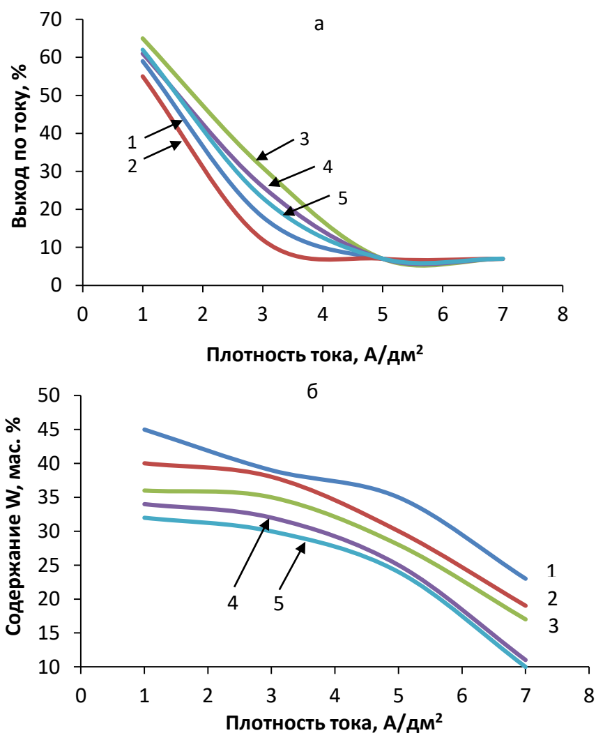
Рисунок 3.39 – Зависимость выхода по току (а) и содержания вольфрама в сплаве Co-W (б) от плотности тока для электролитов с различным соотношением концентраций ионов кобальта и вольфрама, в моль/л: 1) – 0,15/0,35; 2) – 0,2/0,3; 3) – 0,25/0,25; 4) – 0,3/0,2; 5) – 0,35/0,15
