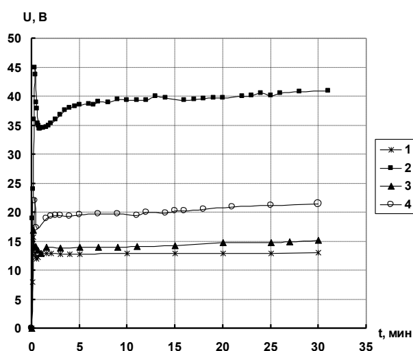
Рисунок 6.2 – Изменение напряжения на ванне при анодировании алюминия А0 в различных электролитах при плотности тока 1 А/дм 2 . Обозначение кривых соответствуют номеру электролита в таблице 6.2
