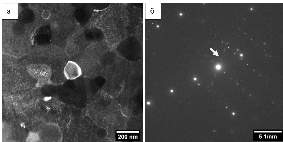
Рисунок 3.35 – Дисперсные частицы NiW в покрытии Ni-44 мас. % W после термообработки при 750 °С в течение 5 ч: а) темнопольное изображение б) электронограмма от частиц. Стрелкой указан рефлекс (0 1 1) NiW
