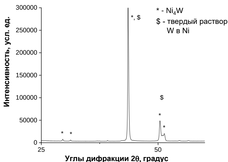
Рисунок 3.22 – Рентгеновская дифрактограмма покрытия Ni-40 мас. % W после съемки ДСК-кривой с разверткой температуры до 1000 °С
