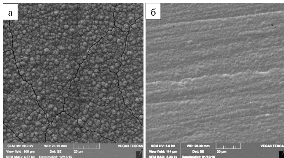
Рисунок 4.4 – Микроструктура поверхности покрытия, осажденного из пиррофосфатного электролита, с концентрацией \text{NaH}_2\text{PO}_2 0,20 моль/л (а) и 0,10 моль/л (б) при плотности тока 4 А/дм 2 . Содержание фосфора 12,0 и 9,9 % соответственно
