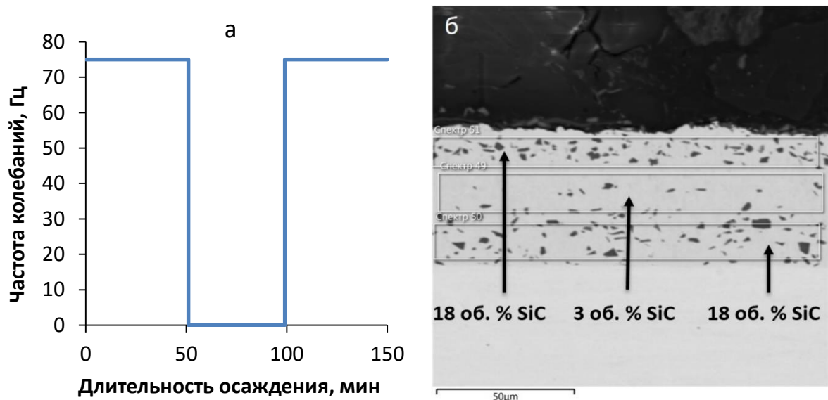
Рисунок 5.40 – Осаждение покрытия Ni-SiC со слоистым распределением частиц SiC: а) график изменения частоты колебаний во времени; б) поперечное сечение покрытия
