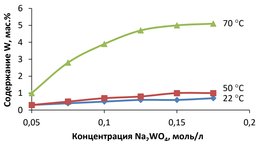
Рисунок 4.11 – Влияние концентрации вольфрамата натрия в электролите на содержание вольфрама в сплаве Ni-P-W при плотности тока 5 А/дм 2 и различных температурах.
