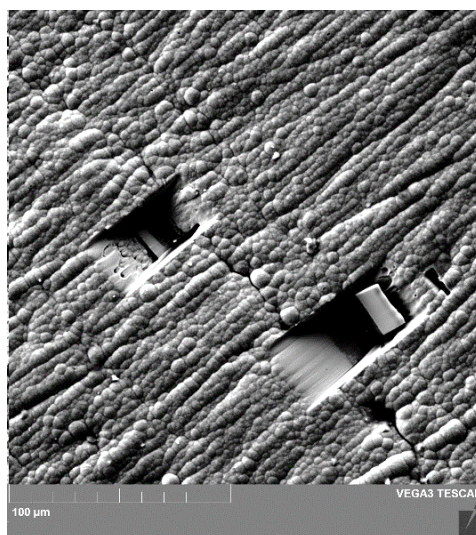
Рисунок 2.7 – Поверхность образца покрытия Ni-44 мас. % W после извлечения ламелей для ПЭМ
