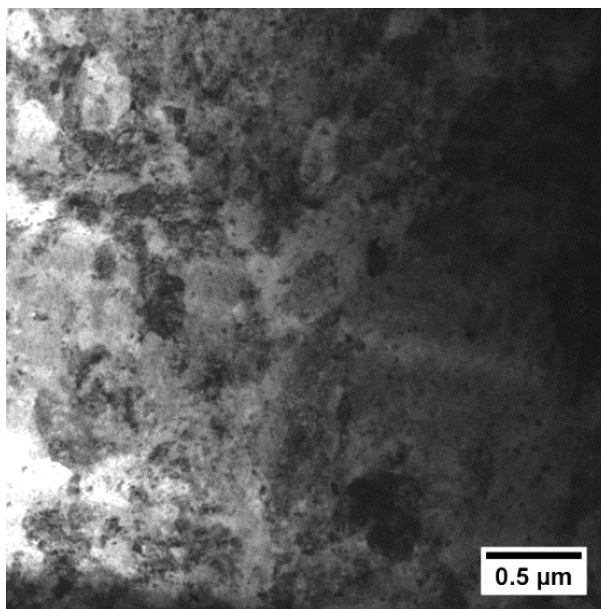
Рисунок 4.20 – Микроструктура покрытия Ni-P-W, термообработанного при 350 °С в течение 3 ч, полученный с помощью просвечивающего электронного микроскопа:
