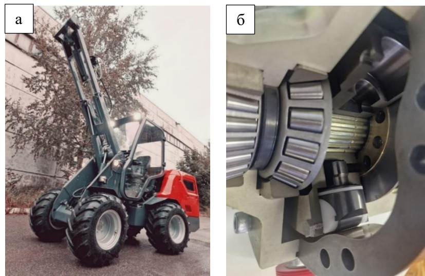
Рисунок 7.5 – Опытный образец мини-трактора производства ООО «Невский инструментальный завод» (а) и демонстрационный гидромотор с открытым кожухом (б)
