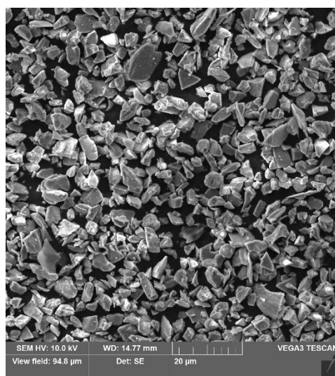
Рисунок 5.1 – Форма частиц порошка карбида кремния фракции М5
