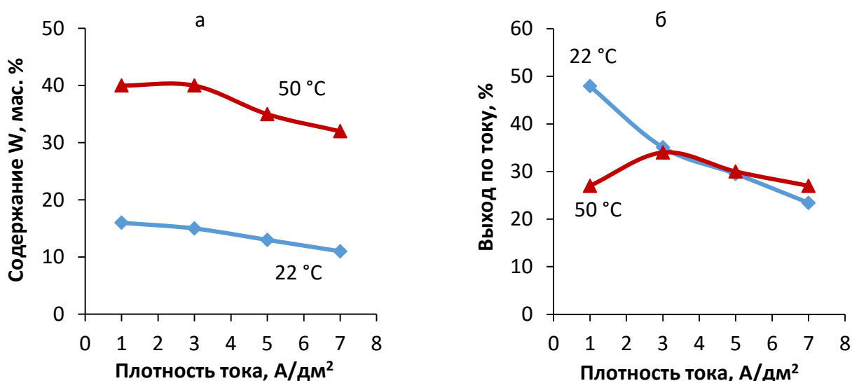
Рисунок 3.6 – Зависимости содержания вольфрама (а) и выхода по току (б) при осаждении покрытия Ni-W от плотности тока при различной температуре
