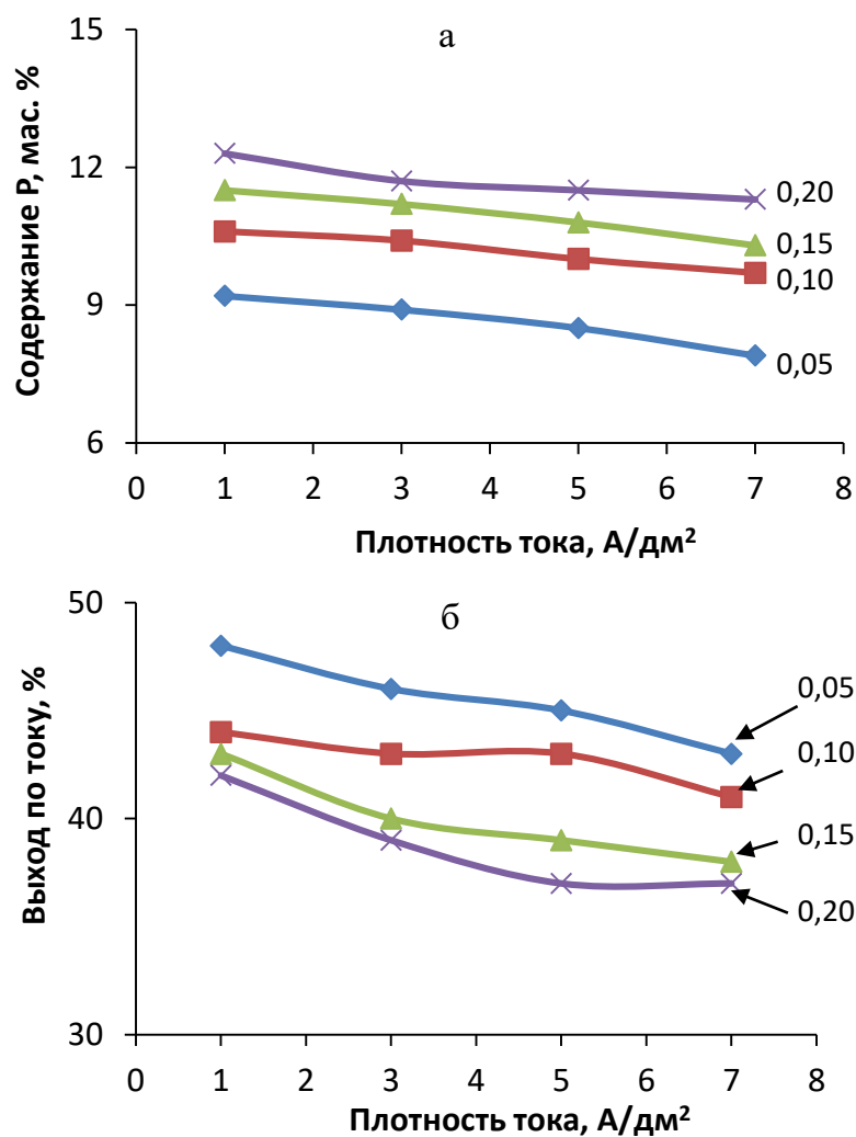
Рисунок 4.6 – Влияние концентрации \text{NaH}_2\text{PO}_2 (в моль/л) в цитратном электролите на содержание фосфора в покрытии Ni-P (а) и его выход по току (б)
