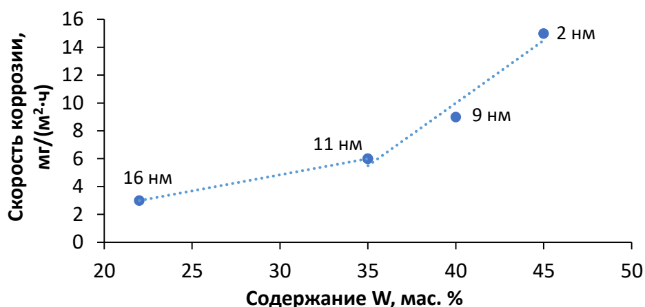
Рисунок 3.15 – Зависимость скорости коррозии сплава Ni-W от содержания вольфрама
