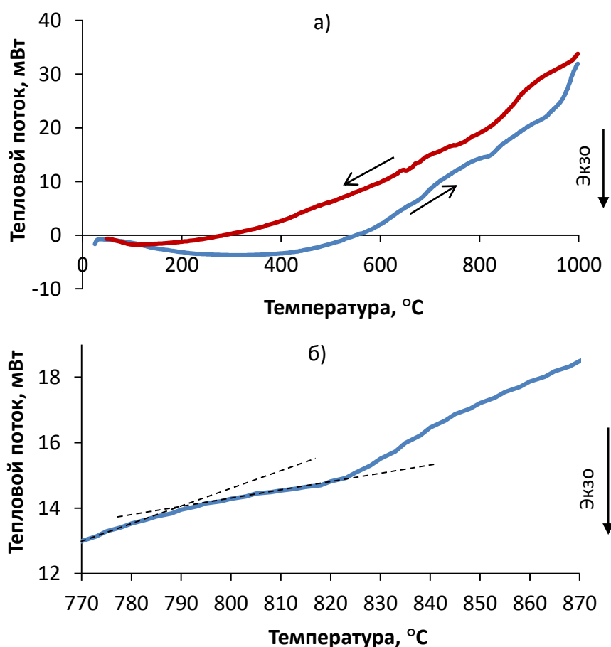
Рисунок 3.20 – Результаты дифференциальной сканирующей калориметрии образца Ni – 40 мас. % W: а) общий вид кривых; б) экзотермический пик кристаллизации
