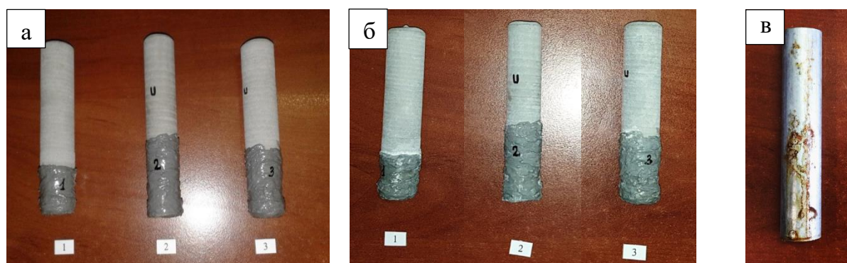
Рисунок 6.14 – Результаты коррозионных испытаний композиционного покрытия Al/ \alpha -Al 2 O 3 -МДО в камере соляного тумана в течение 1000 ч: а) до испытаний; б) после испытаний; в) образец-свидетель без покрытия после испытаний
