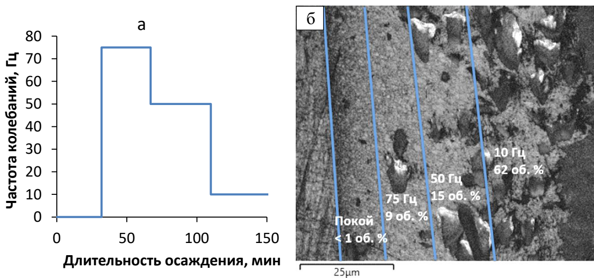
Рисунок 5.41 – Осаждение покрытия Ni-алмаз с градиентным распределением частиц: а) график изменения частоты колебаний во времени; б) поперечное сечение покрытия в режиме контраста полос Кикучи
