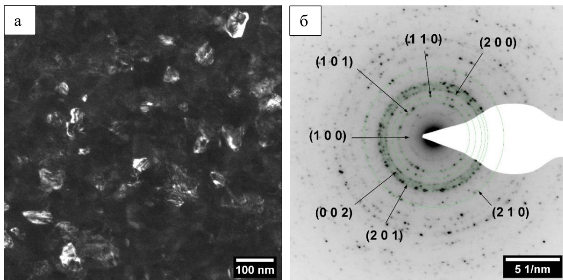
Рисунок 3.51 – Микроструктура покрытия Co-W после термообработки при 750 °С в течение 5 ч: а) темнопольное изображение; б) электронограмма
