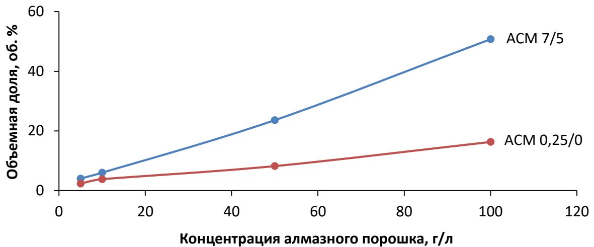
Рисунок 5.34 – Зависимость объемной доли алмаза в композиционном покрытии от его концентрации в электролите
