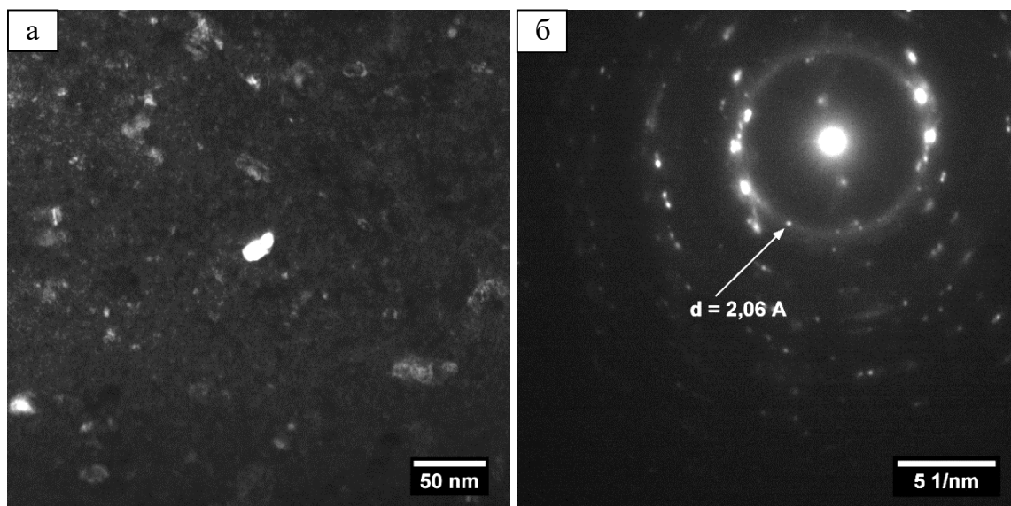
Рисунок 4.21 – Матрица покрытия Ni-P-W после термической обработки при 350 °С в течение 3 ч: а) темнопольное изображение; б) электронограмма
