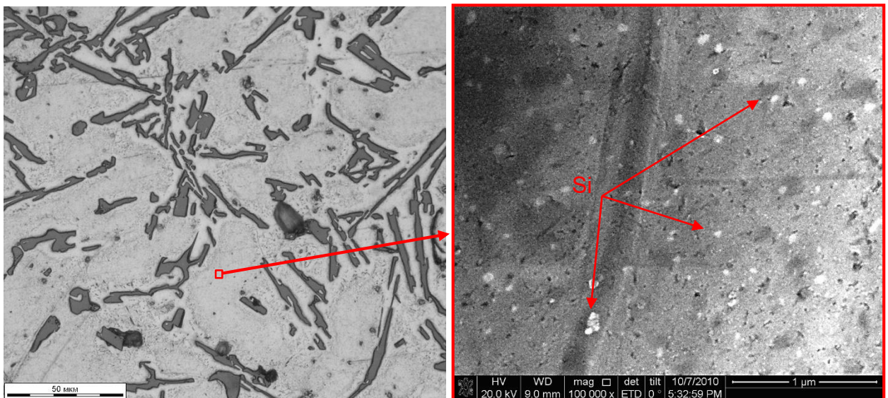
Рисунок 6.5 – Строение анодного оксидного покрытия через 15 с после включения тока (начальная стадия формирования)
