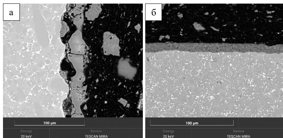
Рисунок 7.9 – Сравнение микроструктуры покрытий, полученных микродуговым оксидированием (а) и анодированием (б) на сплаве ADC12
