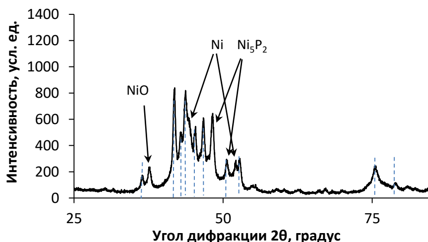
Рисунок 4.18 – Рентгеновская дифрактограмма покрытия Ni-P-W после термообработки в течение 6 ч при 350 °С. Штриховыми линиями отмечено положение рефлексов фазы \text{Ni}_3\text{P}
