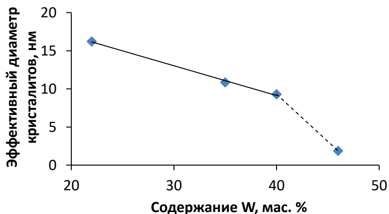
Рисунок 3.12 – Результаты расчета эффективного диаметра кристаллитов по Шерреру для сплавов Ni-W различного химического состава
