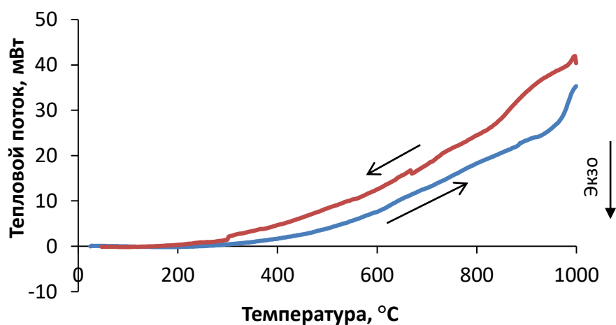
Рисунок 3.19 – Результаты дифференциальной сканирующей калориметрии образца покрытия Ni – 35 мас. % W
