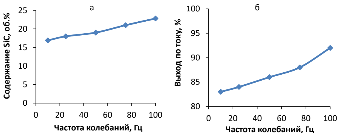
Рисунок 5.17 – Влияние частоты колебаний на объемную долю карбида кремния (а) и выход по току (б) покрытия Ni-SiC при осаждении из электролита с субмикронным порошком
