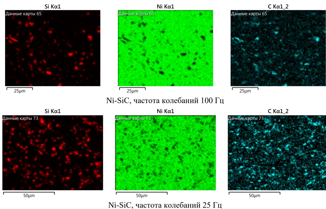
Рисунок 5.9 – Карты элементов для образцов покрытия Ni-SiC, полученных при различных частотах колебаний вибрационной мешалки
