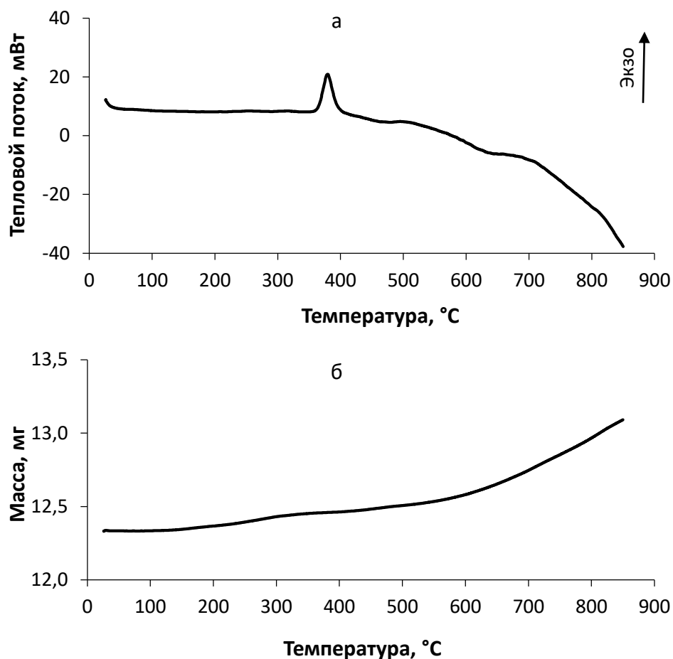
Рисунок 4.15 – Зависимости изменения теплового потока (а) и массы (б) от температуры кривые для образца покрытия Ni-P-W
