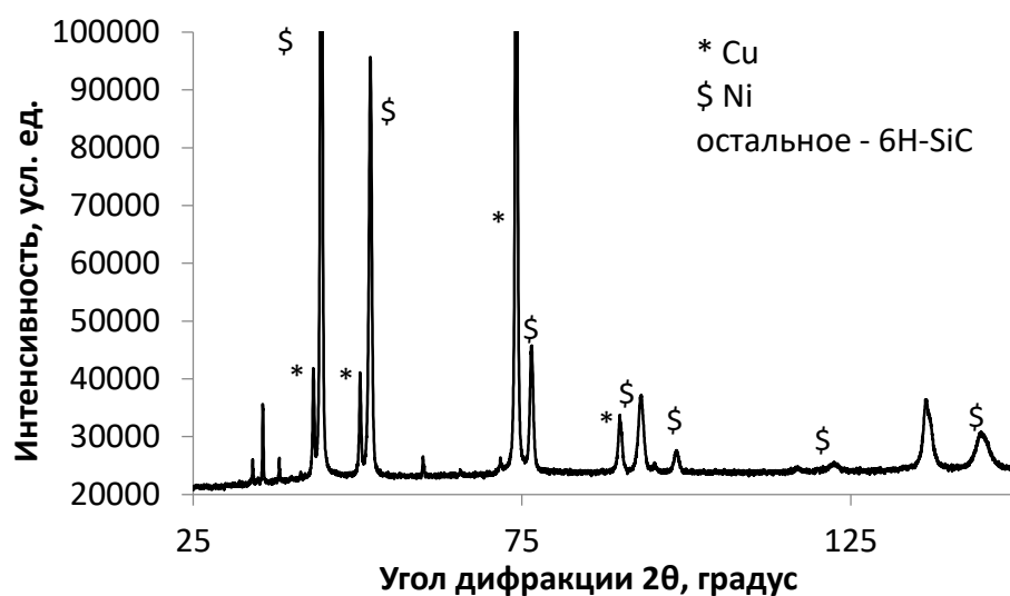
Рисунок 5.7 – Рентгеновская дифрактограмма покрытия Ni-SiC
