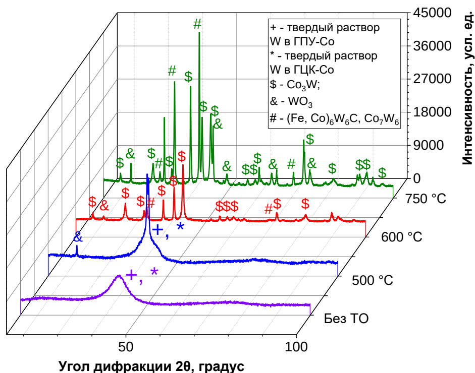
Рисунок 3.48 – Рентгеновские дифрактограммы образцов покрытия Co-45 мас. % W в исходном состоянии (обозначено «Без ТО») и после термообработки в течение 5 ч при различных температурах
