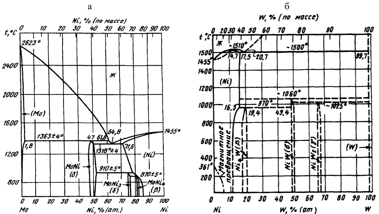
Рисунок 1.4 – Диаграммы состояния Ni-Mo (а) и Ni-W (б) [10].
