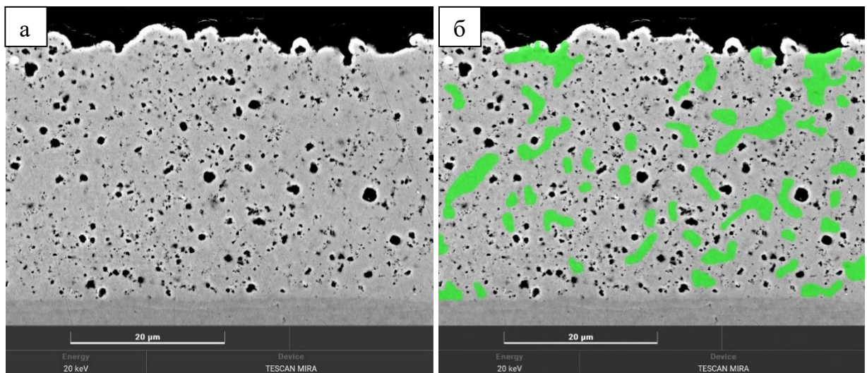
Рисунок 5.24 – Поперечное сечение композиционного покрытия, сформированного при продолжительном осаждении 2,5 ч при плотности тока 2 \text{ А/дм}^2 и частоте колебаний 50 Гц: а) исходное изображение; б) визуализация зон без частиц SiC
