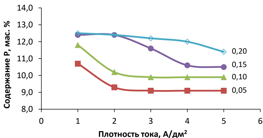
Рисунок 4.3 – Зависимость содержания фосфора в покрытии Ni-P от плотности тока при осаждении из электролитов с различной концентрацией гипофосфита натрия, моль/л
