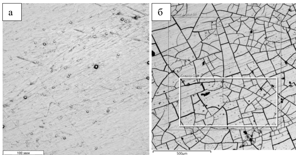
Рисунок 3.41 – Микроструктура поверхности покрытия Co-53 мас. % W: а) свежесозданное покрытие, оптическое изображение; б) разрушение покрытия при вакуумировании в электронном микроскопе
