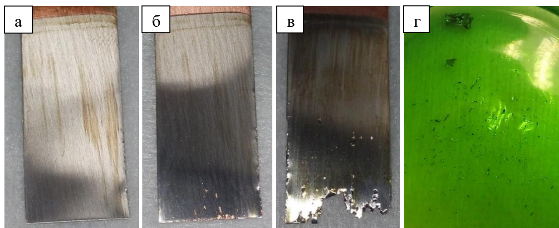
Рисунок 3.17 – Коррозия медных образцов с покрытием Ni-45 мас. % W толщиной 3 мкм в 70 %-ной \text{HNO}_3 при различных временах экспозиции: а) 5 с; б) 90 с; в) 300 с; г) фрагменты покрытия в азотной кислоте
