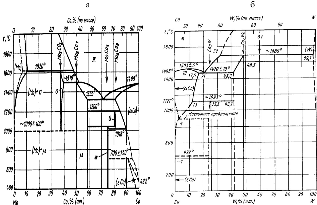
Рисунок 1.3— Диаграммы состояния Mo-Co (а) и Co-W (б) [25]
