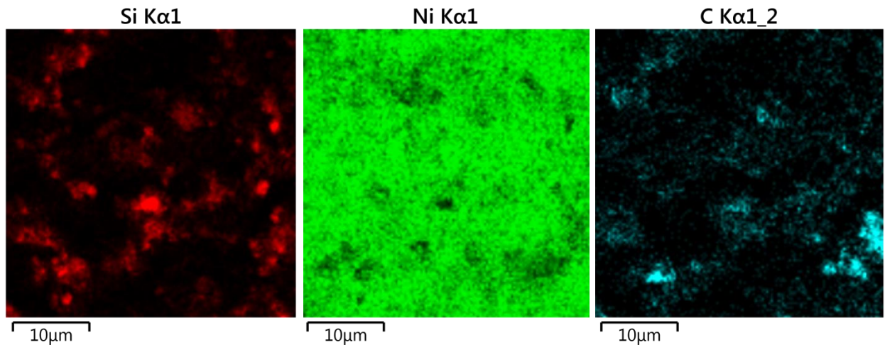
Рисунок 5.22 – Карты распределения элементов по поверхности покрытия Ni-SiC, осажденного при частоте 50 Гц и амплитуде колебаний 1 мм. Содержание SiC – 19 об. %.
