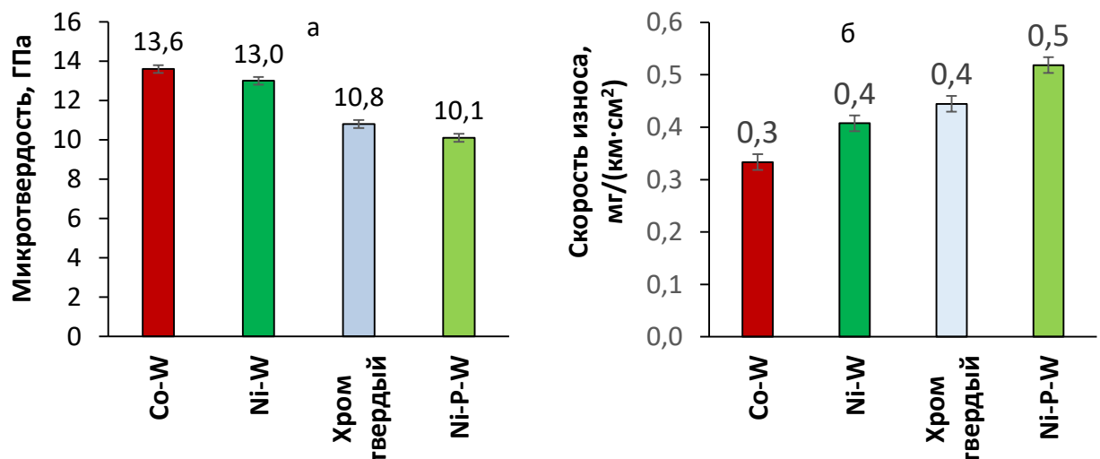
Рисунок 7.2 – Сравнение микротвердости (а) и скорости износа в паре трения с корундом (б) кристаллизационных композиционных покрытий
