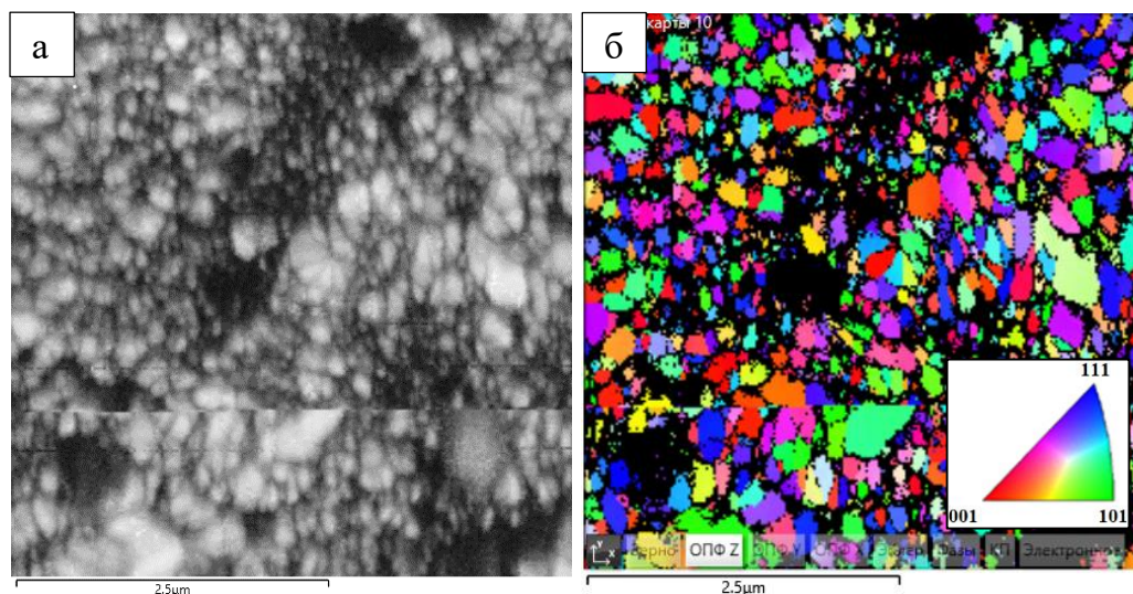
Рисунок 5.27 – Структура никелевой матрицы композиционного покрытия Ni-SiC, полученного с порошком субмикронного размера: а) режим контраста полос Кикучи; б) карта ориентировок кристаллитов
