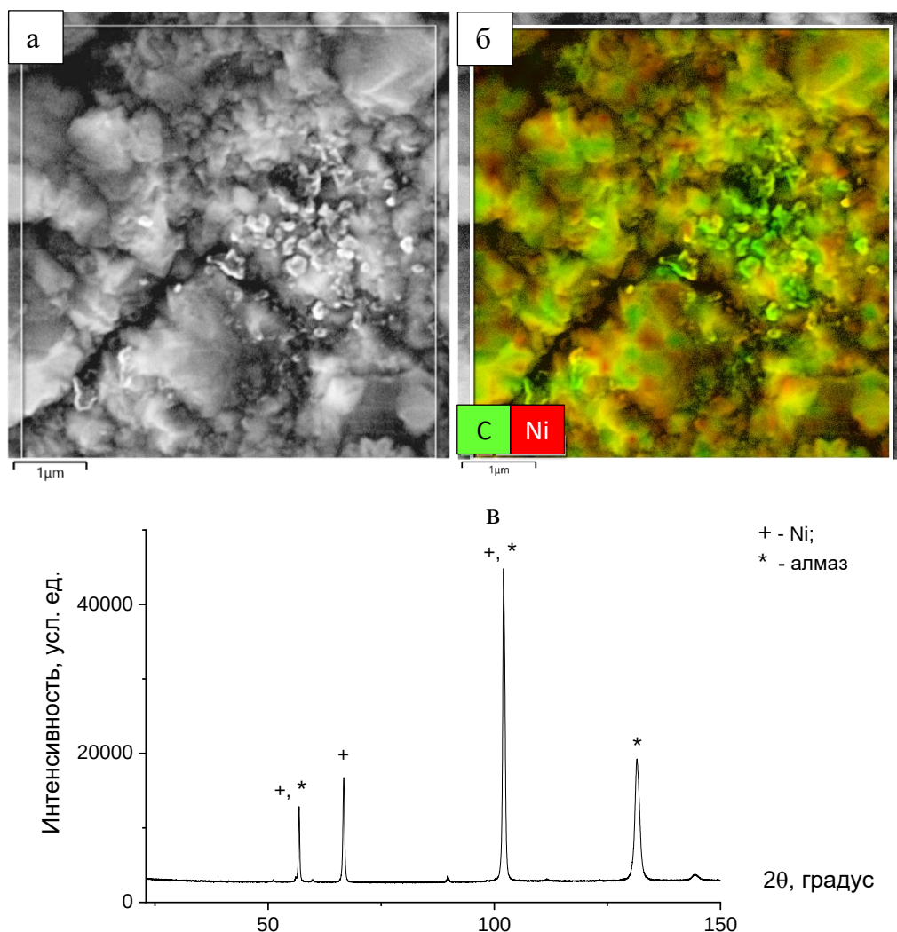
Рисунок 5.33 – Скопление частиц алмаза в покрытии никель-алмаз, полученном с порошком алмаза АСМ 0,25/0 (а), и его многослойное изображение с картой элементов (б); дифрактограмма образца покрытия (в)
