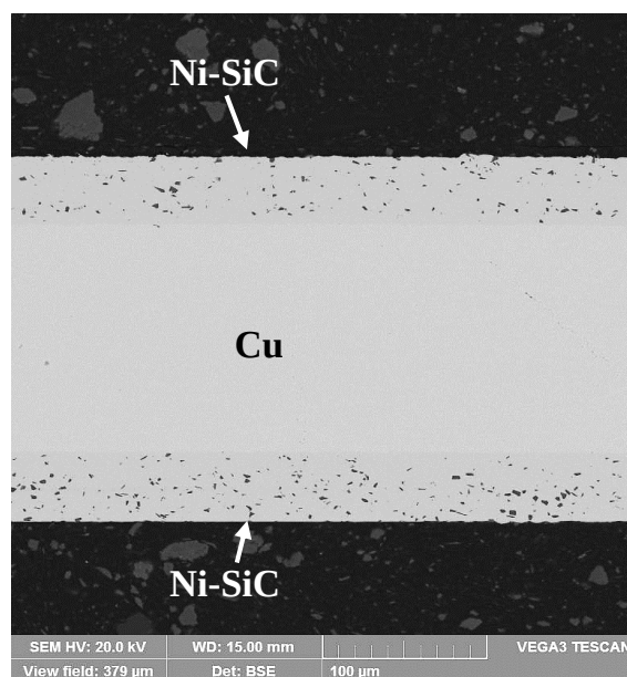
Рисунок 5.4 – Поперечное сечение образца с покрытием Ni-SiC, полученного в условиях вибрационного перемешивания
