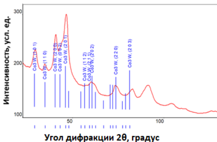
Рисунок 3.52 – Анализ электронограммы покрытия Co-W после термообработки при 750 °С в течение 5 ч
