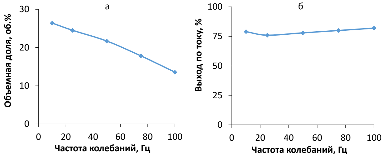
Рисунок 5.10 – Влияние частоты колебаний на объемное содержание карбида кремния размерности М5 (а) и выход по току композиционного покрытия (б)
