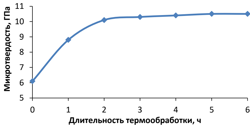
Рисунок 4.17 – Зависимость микротвердости покрытия Ni-P-W от продолжительности термообработки при 350 °С
