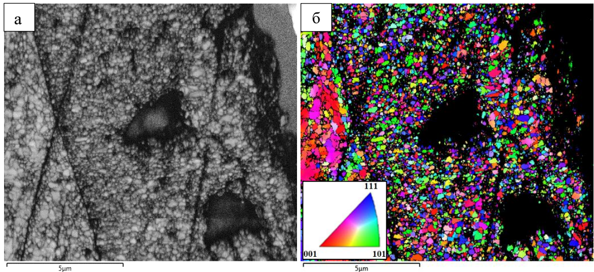
Рисунок 5.37 – Микроструктура никелевой матрицы композиционного покрытия Ni-алмаз, полученного с порошком АСМ 7/5: а) режим контраста полос Кикучи; б) карта ориентировок кристаллитов
