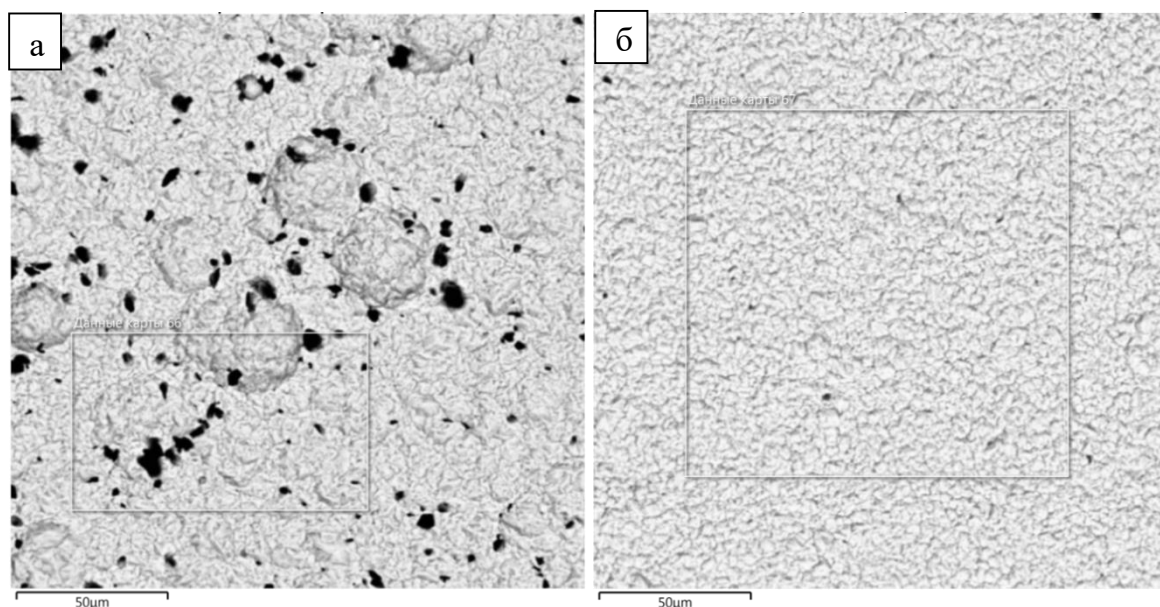
Рисунок 5.3 – Микроструктура поверхностей образца с композиционным покрытием Ni-SiC, осажденного в отсутствие вибрации при плотности тока 3 \text{ А/дм}^2 : а) поверхность, обращенная к зеркалу электролита; б) поверхность, обращенная к дну ванны
