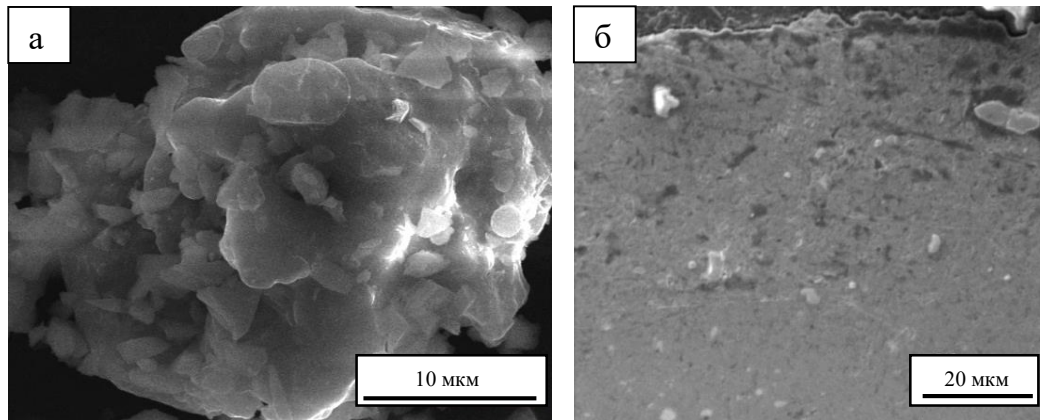
Рисунок 6.12 – Структура частицы композиционного порошка Al-SiC (а) и микроструктура покрытия Al-SiC (б)
