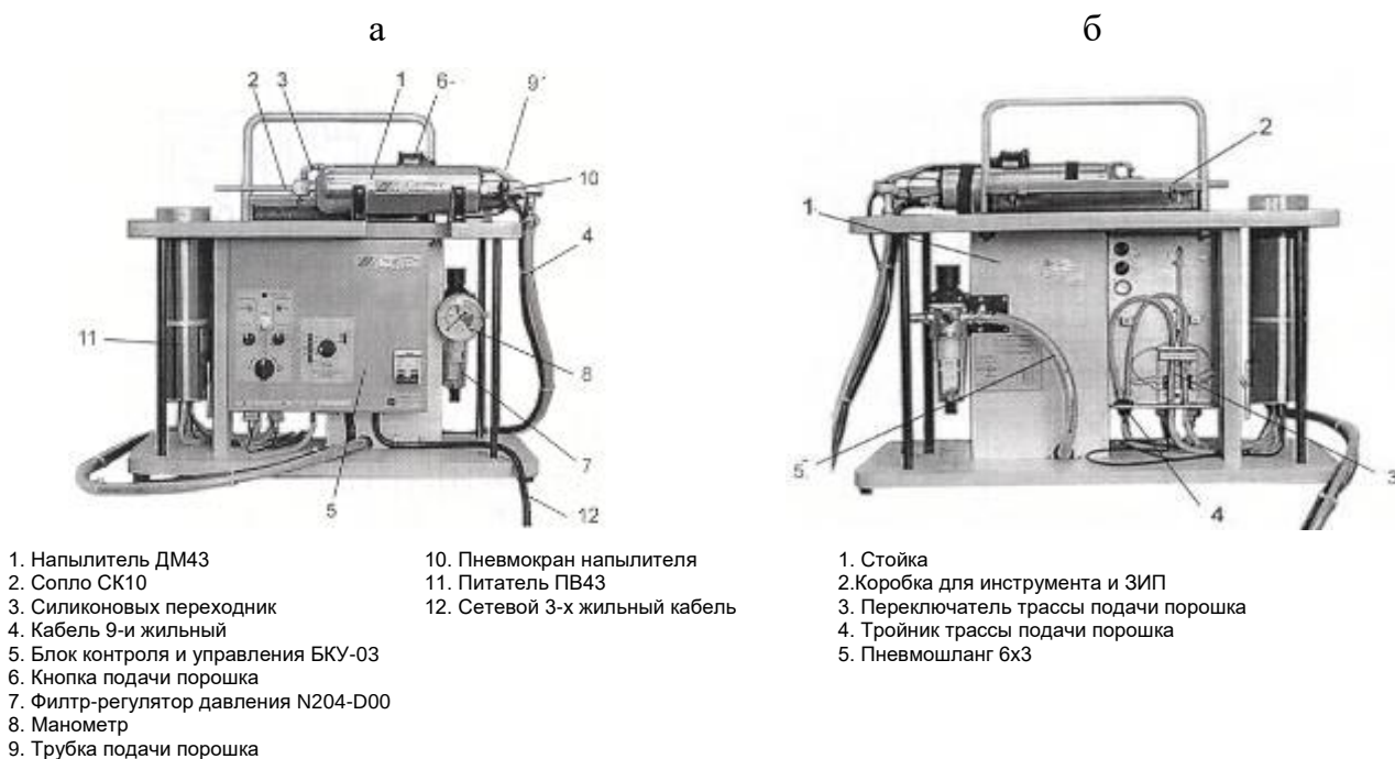
Рисунок 2.5 – Внешний вид установки «Димет-403»: а) лицевая сторона; б) обратная сторона
