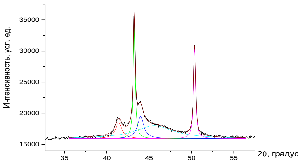
Рисунок 2.6 – Пример анализа дифрактограммы для покрытия Co-W.
