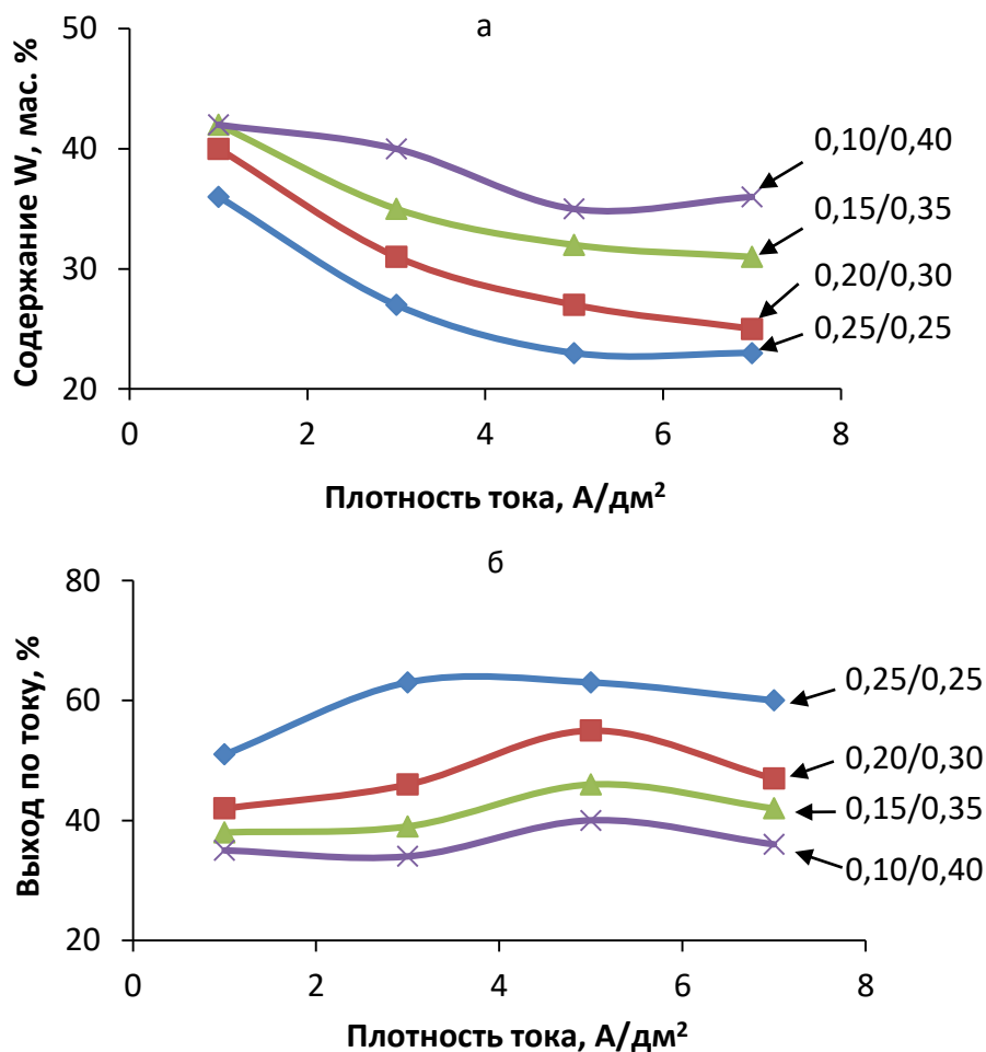
Рисунок 3.9 – Влияние соотношения концентраций ионов никеля и вольфрама на состав покрытия (а) и выход по току (б) при суммарной концентрации ионов никеля и вольфрама 0,5 моль/л, избытке цитрат-ионов 0,3 моль/л и рН 8,0 и температуре электролита 50 °С
