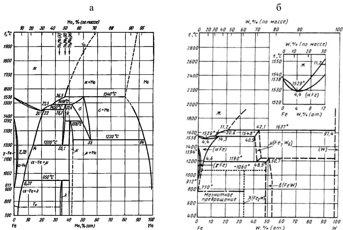
Рисунок 1.2 – Диаграммы состояния сплава Fe-Mo [26] (а) и Fe-W [25] (б)
