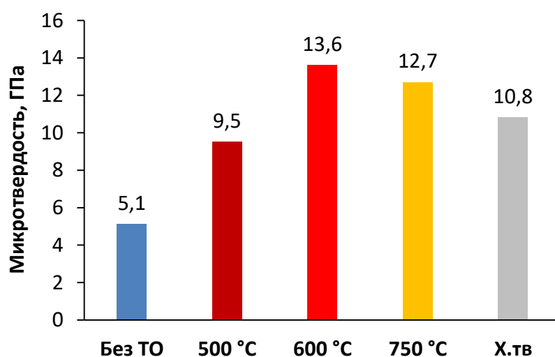
Рисунок 3.49 – Влияние температуры термообработки покрытий Co-45 мас. % W на микротвердость. Длительность термообработки 5 ч. Данные приведены в сравнении с покрытием «хром твердый» (Х.тв)
