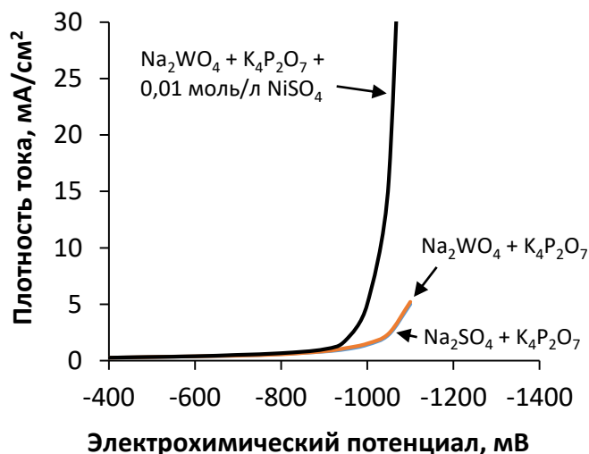
Рисунок 3.3 – Катодные поляризационные кривые на графитовом электроде в электролитах различного состава
