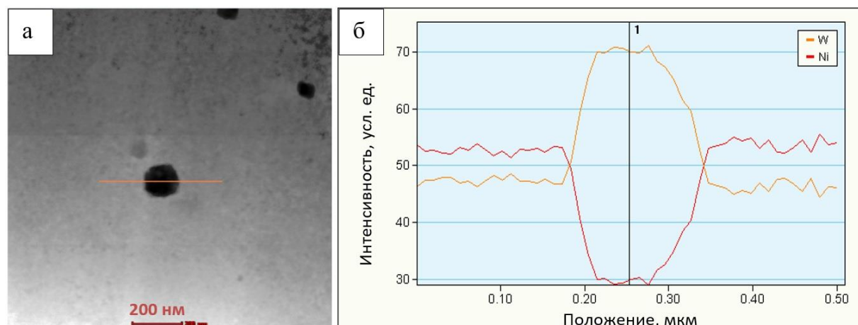
Рисунок 3.30 – Распределение элементов вдоль линии, пересекающей частицу NiW: а) изображение частицы; б) измерение элементного состава
