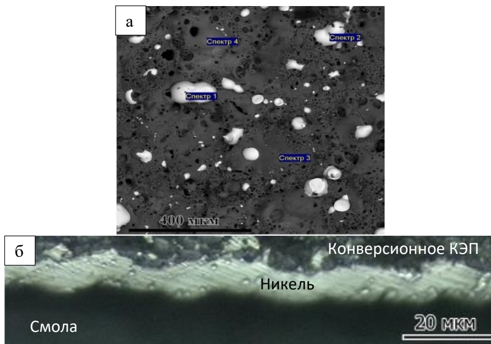
Рисунок 6.16 – Микроструктура композиционного покрытия типа «оксидная матрица – никель»: а) структура поверхности на финальной стадии заполнения пор; б) поперечное сечение покрытия с внешним металлическим слоем
