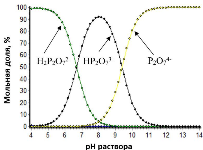
Рисунок 3.2 – Распределение протонированных форм дифосфат-иона в зависимости от pH. Расчет по константам диссоциации по данным [334, с. 79]
