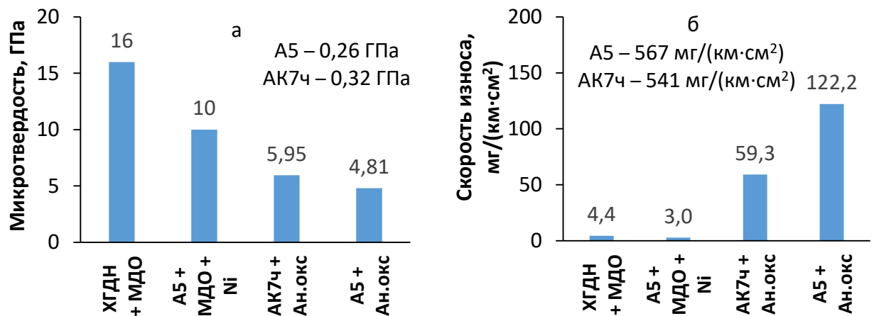
Рисунок 7.4 – Сравнение микротвердости (а) и скорости изнашивания (б) конверсионных покрyтий
