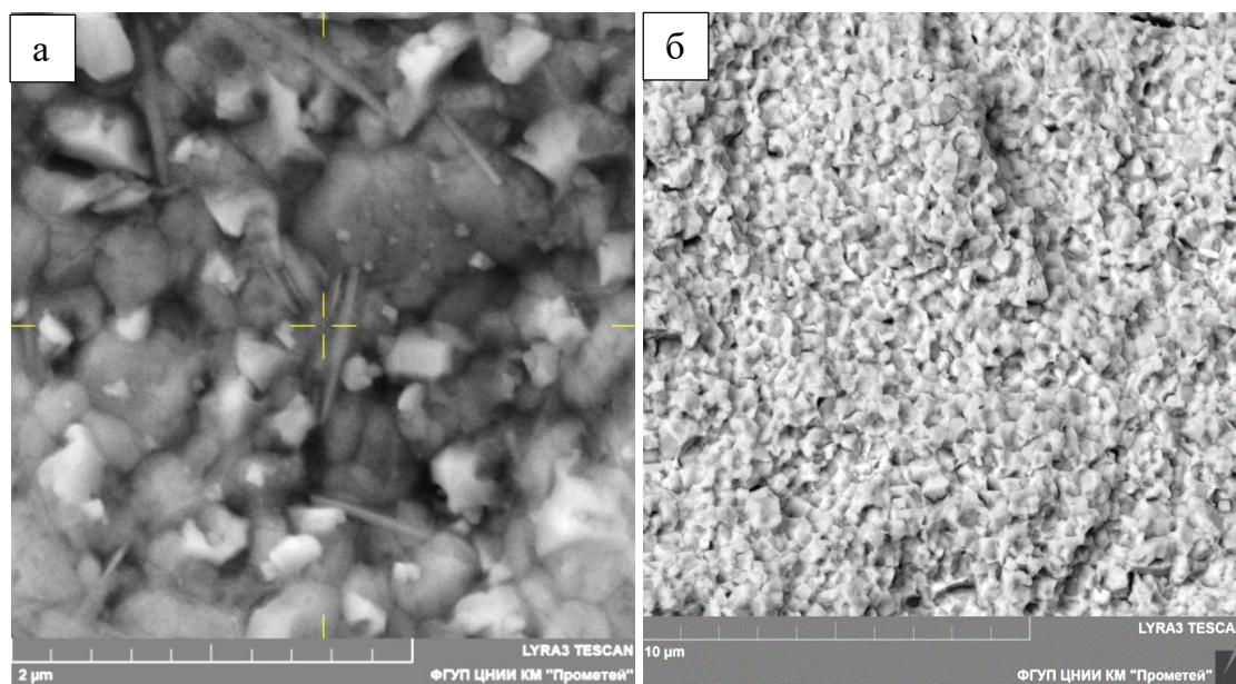
Рисунок 3.21 – Образец электроосажденного сплава Ni – 40 % W после снятия ДСК-кривой с разверткой температуры до 1000 °С: а) микроструктура поверхности; б) микроструктура излома
