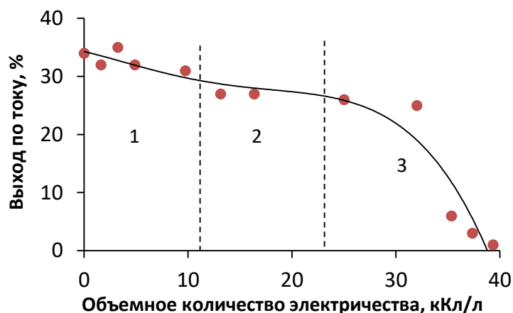
Рисунок 3.7 – Зависимость выхода по току при осаждении сплава Ni-W от количества электричества, пропущенного через ванну без применения мембранного электролизера. Плотность тока 3 А/дм 2
