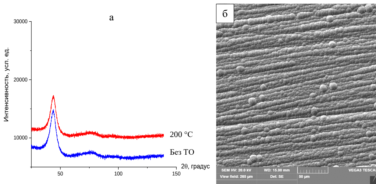
Рисунок 3.46 – Состояние образца с покрытием из сплава Co-45 мас. % W после термообработки при 200 °C в течение 5 ч: дифрактограммы покрытий (а) и электронное изображение поверхности (б)
