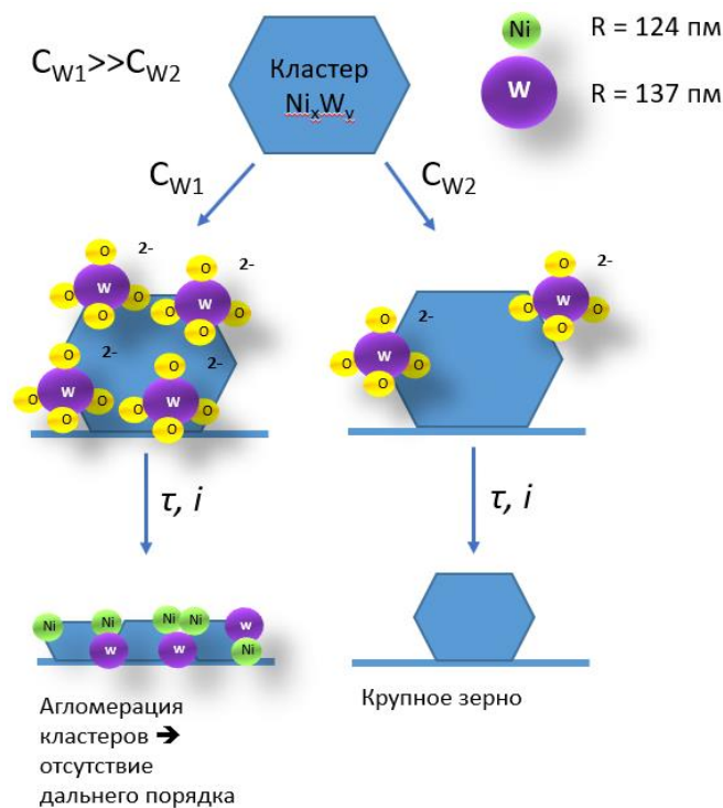
Рисунок 3.5 – Схема роста покрытий Ni-W:
