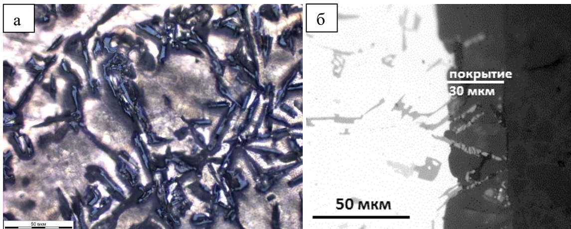
Рисунок 6.9 – Микроструктура поверхности (а) и поперечное сечение (б) конверсионного КЭП на сплаве АК7ч, полученного анодированием в течение 30 мин в электролите № 3 при плотности тока 3 А/дм 2
