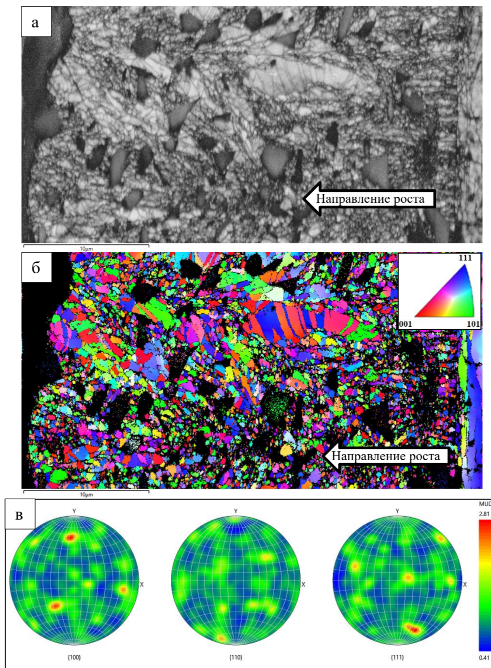
Рисунок 5.26 – Микроструктура композиционного покрытия Ni-SiC с фракцией карбида кремния M5: а) микроструктура, полученная в режиме контраста полос Кикучи; б) карта ориентировок кристаллов; в) полюсные фигуры
