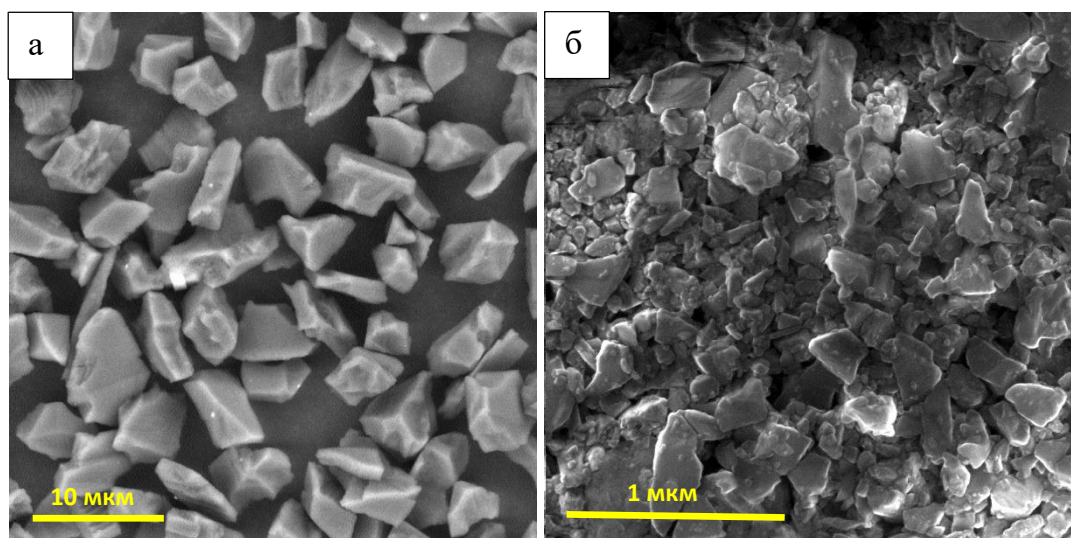
Рисунок 5.30 – Электронное изображение алмазных порошков: а) АСМ 7/5; б) субмикронный порошок АСМ 0,25/0
