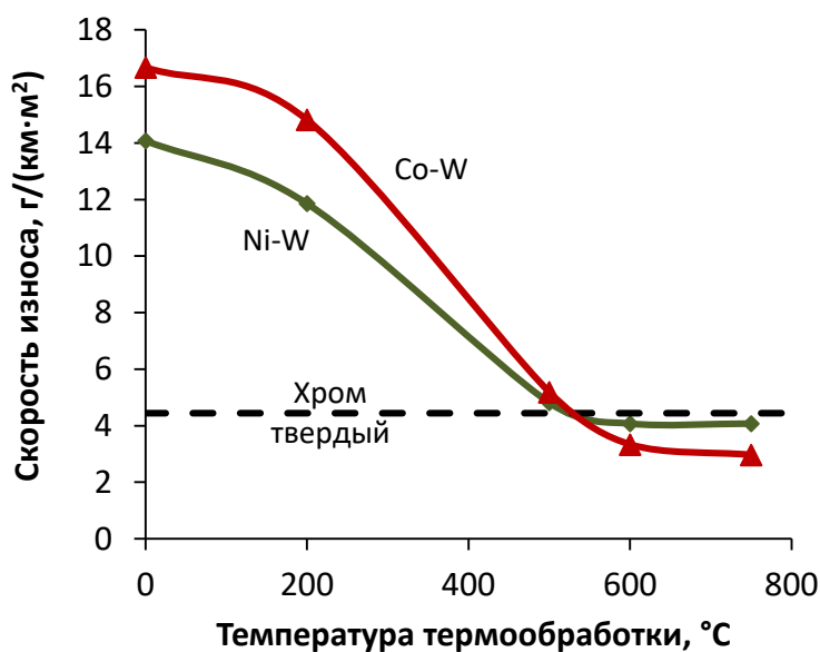
Рисунок 3.56 – Влияние температуры термообработки на скорость изнашивания покрытий Ni-W и Co-W в паре трения скольжения с корундом. Длительность термообработки 5 ч
