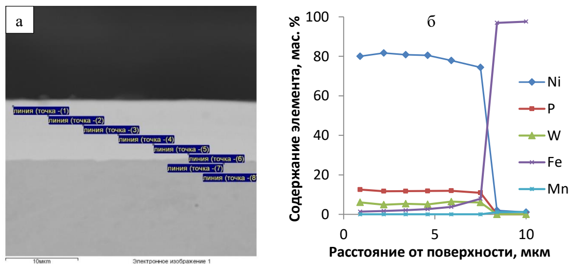
Рисунок 4.19 – Расположение точек сканирования химического состава покрытия термообработанного Ni-P-W (а) и градиент химического состава по толщине покрытия (б)
