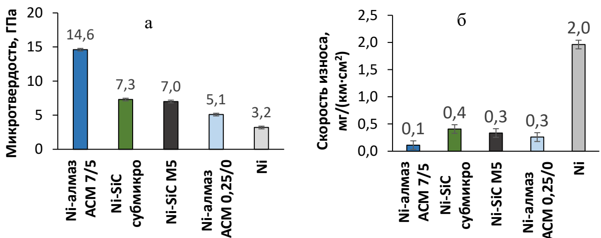
Рисунок 7.1 – Сравнение микротвердости (а) и скорости износа (б) классических КЭП, полученных в условиях виброперемешивания, с гальваническим никелем по ГОСТ 9.305
