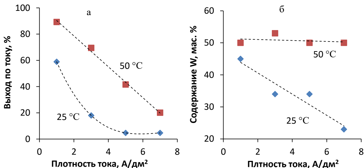
Рисунок 3.40 – Зависимости выхода по току (а) и содержания вольфрама (б) от плотности тока для электролита осаждения сплава Co-W с соотношением концентраций ионов кобальта и вольфрама (в моль/л) 0,15/0,35
