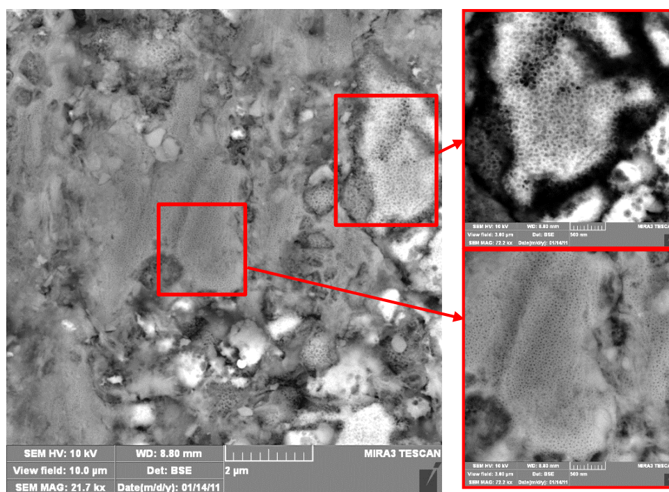
Рисунок 6.6 – Структура анодного оксидного покрытия через 5 мин после включения тока (стадия формирования пористого слоя)
