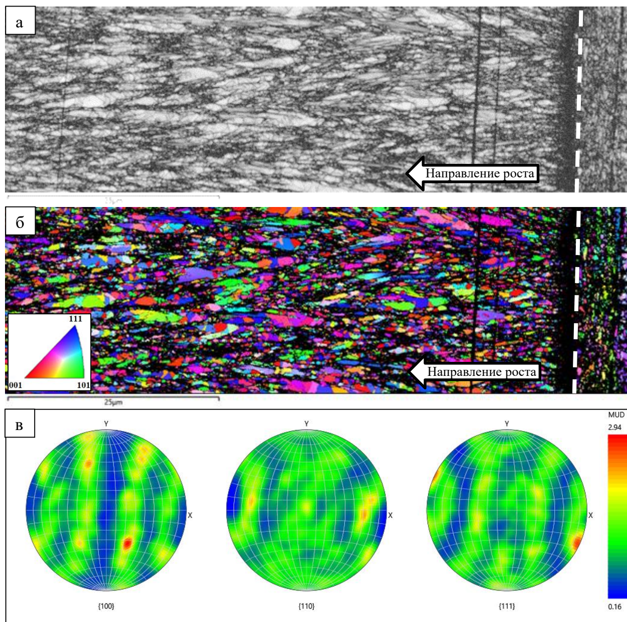
Рисунок 5.25 – Микроструктура никелевого покрытия: а) микроструктура, полученная в режиме контраста полос Кикучи; б) карта ориентировок кристаллов; в) полюсные фигуры
