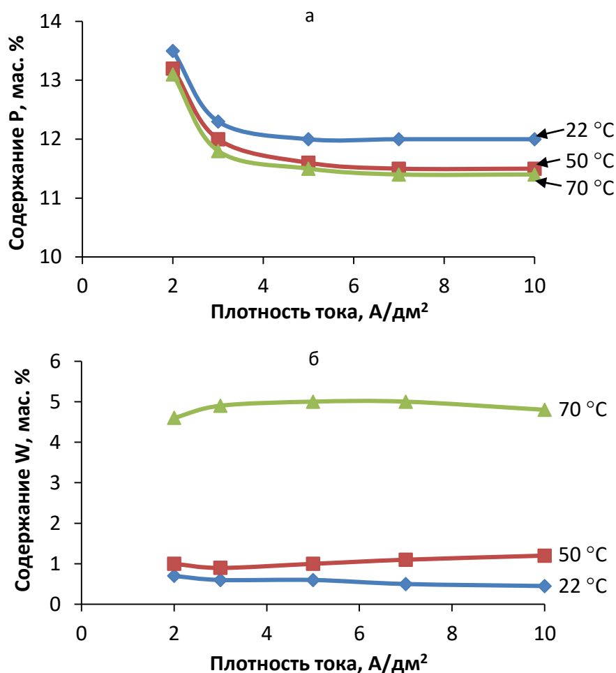
Рисунок 4.12 – Влияние плотности тока и температуры электролита на химический состав покрытия: а) содержание фосфора; б) содержание вольфрама.
