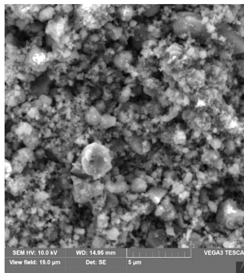
Рисунок 5.14 – Форма частиц субмикронного порошка карбида кремния
