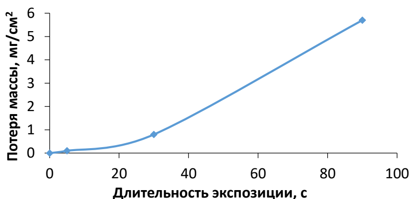
Рисунок 3.16 – Изменение массы во времени медного образца с покрытием Ni-45 мас. % W при выдержке в 70 %-ной азотной кислоте
