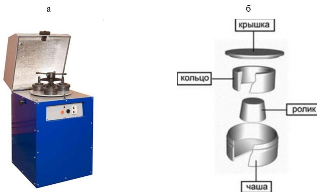
Рисунок 2.4 – Вибрационный чашечный истиратель ИВЧ-3: а) внешний вид; б) схема расположения рабочих элементов истирателя
