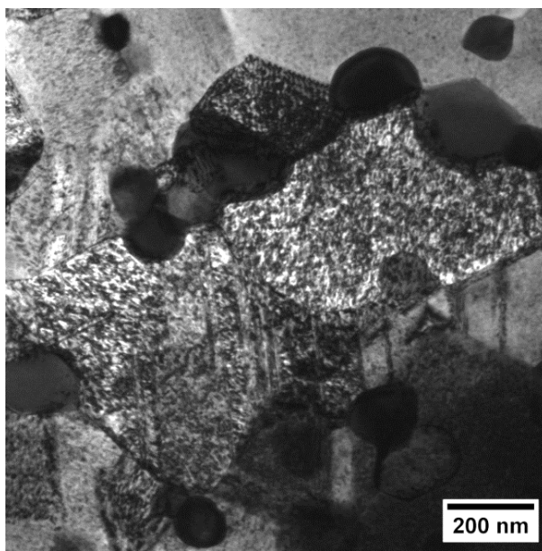
Рисунок 3.32 – Светлопольное изображение микроструктуры покрытия Ni-44 мас. % W, термообработанного при 750 °С в течение 5 ч
