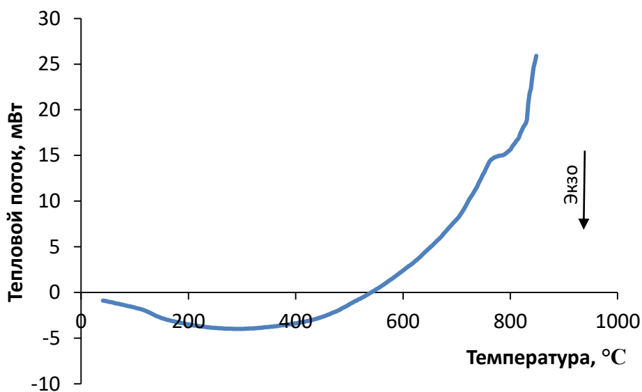
Рисунок 3.23 – Результаты дифференциальной сканирующей калориметрии образца покрытия Ni-44 мас. % W
