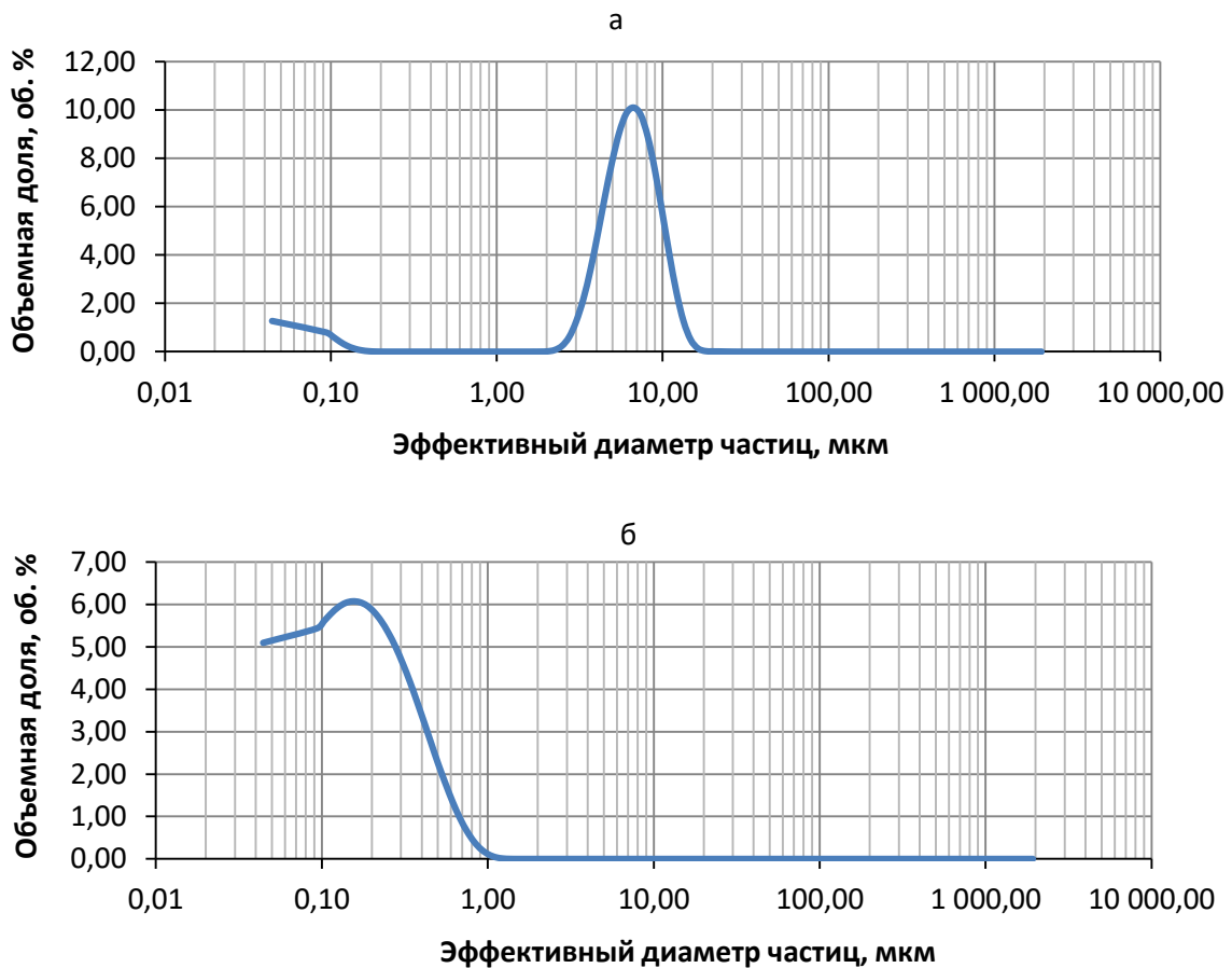
Рисунок 5.29 – Гранулометрический состав алмазных порошков: а) порошок АСМ 7/5; б) субмикронный порошок АСМ 0,25/0
