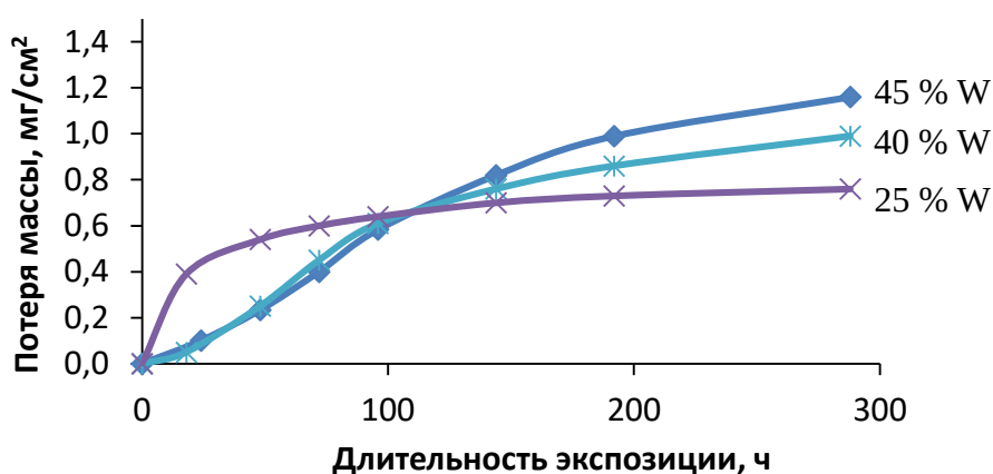
Рисунок 3.43 – Зависимость потери массы образцов покрытий Co-W с различным содержанием вольфрама (в мас. %) от времени коррозии в 3,5 %-ном растворе NaCl
