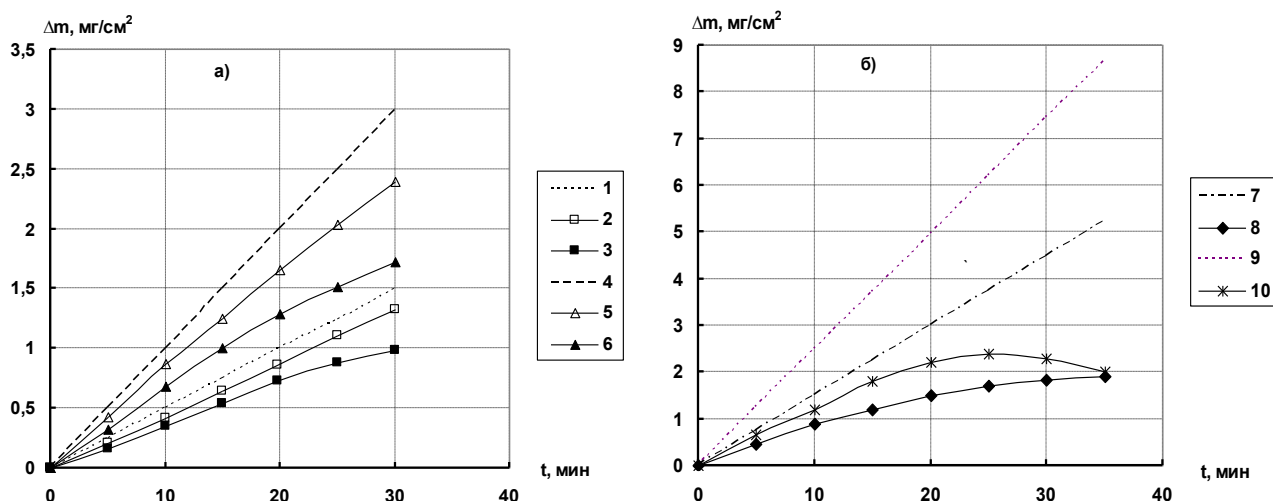
Рисунок 6.8 – Изменение во времени массы алюминия (кривые 2 и 5) и сплава АК7ч (кривые 3, 6, 8 и 10) при анодировании в электролите 3 при плотности тока: кривые 1, 2, 3 – 1 А/дм 2 ; кривые 4, 5, 6 – 2 А/дм 2 ; кривые 7, 8 – 3 А/дм 2 ; кривые 9, 10 – 5 А/дм 2 . Пунктирные кривые 1, 4, 7 и 9 – теоретические кривые изменения массы во времени при плотности тока соответственно 1 А/дм 2 , 2 А/дм 2 , 3 А/дм 2 и 5 А/дм 2
