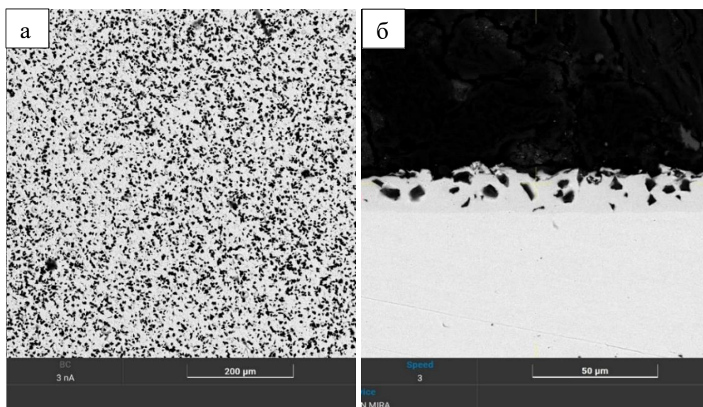
Рисунок 5.36 – Микроструктура никель-алмазного покрытия, полученного с использованием алмазного порошка АСМ 7/5. Объемная доля 23,6 %: а) поверхность; б) поперечное сечение
