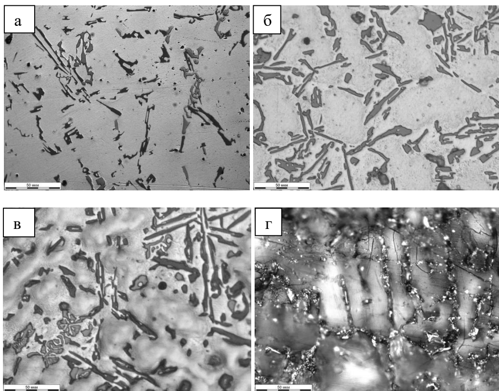
Рисунок 6.4 – Микрофотографии поверхности полированного образца силумина после анодирования в электролите № 3 при плотности тока 1 \text{ А/дм}^2 в течение различного времени: а) без анодирования; б) 30 с; в) 5 мин; г) 30 мин
