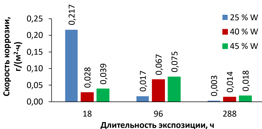
Рисунок 3.44 – Скорость коррозии (дифференциальное значение) покрытий Co-W в различные моменты времени
