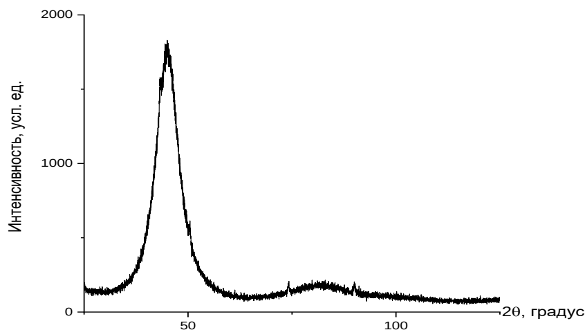
Рисунок 4.8 – Рентгеновская дифрактограмма покрытия Ni-10 % Р, полученного из пирофосфатного электролита
