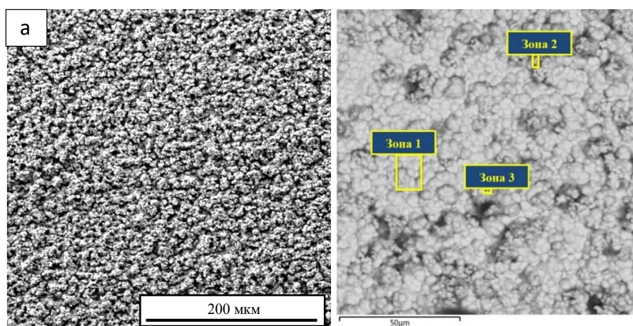
Рисунок 5.21 – Микроструктура поверхности композиционного покрытия Ni-SiC, осажденного при частоте вибрации 50 Гц и амплитуде 1 мм (а) и зоны исследования химического состава структурных элементов покрытия (б)
