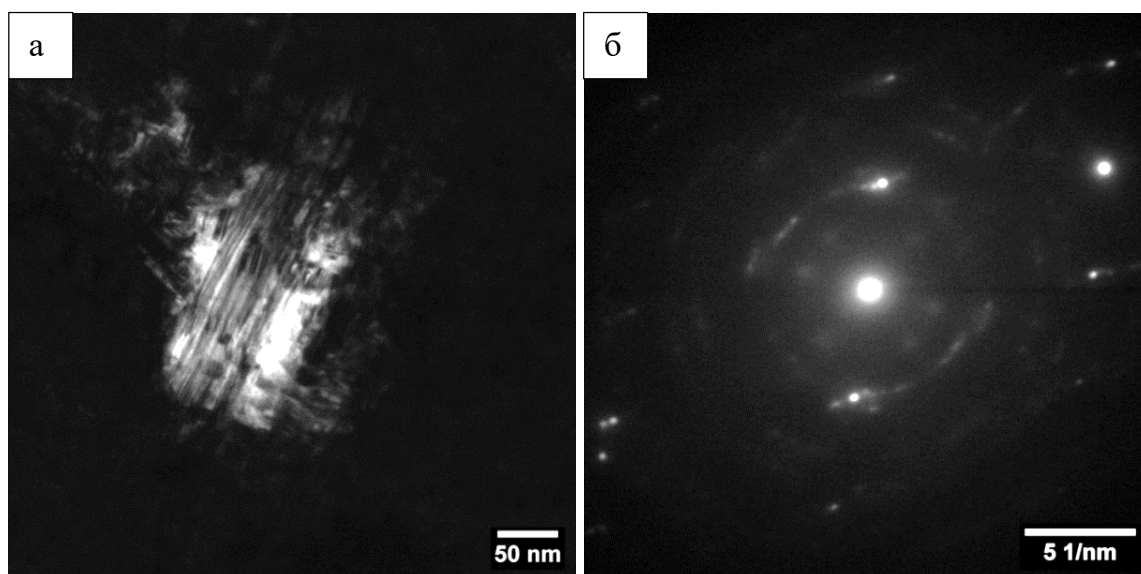
Рисунок 3.31 – Частица интерметаллида \text{Ni}_4\text{W} в образце Ni-44 мас. % W, термообработанного при 600 °C в течение 5 ч: а) темнопольное изображение; б) электронограмма от частицы
