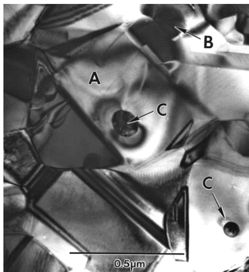
Рисунок 3.36 – Микроструктура покрытия Ni-W после термообработки при температуре 800 °С в течение 24 ч (по данным [178]): А – зерно Ni_4W ; В – выделения NiW ; С – W_{1,3}Ni_{0,24}O_4
