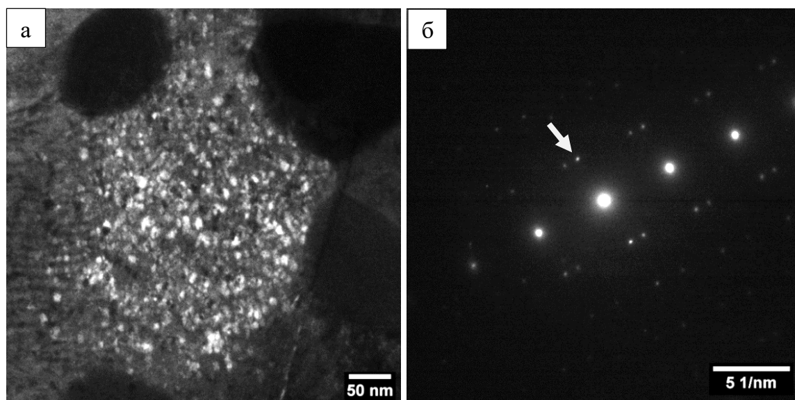
Рисунок 3.34 – Дисперсные частицы \text{Ni}_4\text{W} в зернах твердого раствора: а) темнопольное изображение; б) электронограмма. Стрелкой указан рефлекс (0 1 1) \text{Ni}_4\text{W}
