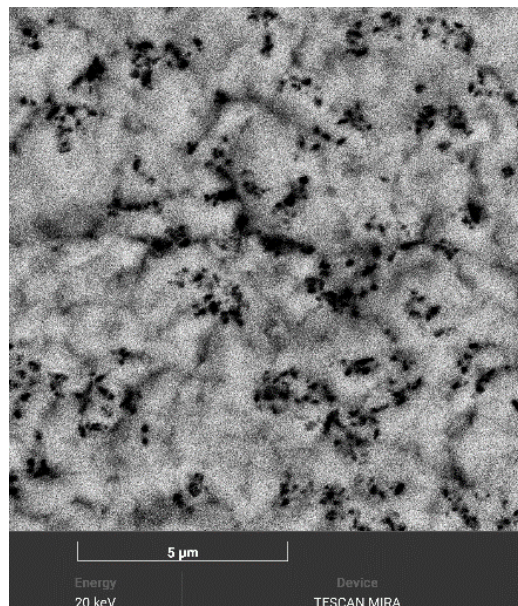
Рисунок 5.32 – Микроструктура поверхности композиционного покрытия Ni-алмаз (АСМ 0,25/0), полученного электроосаждением при вибрационном перемешивании электролита-суспензии
