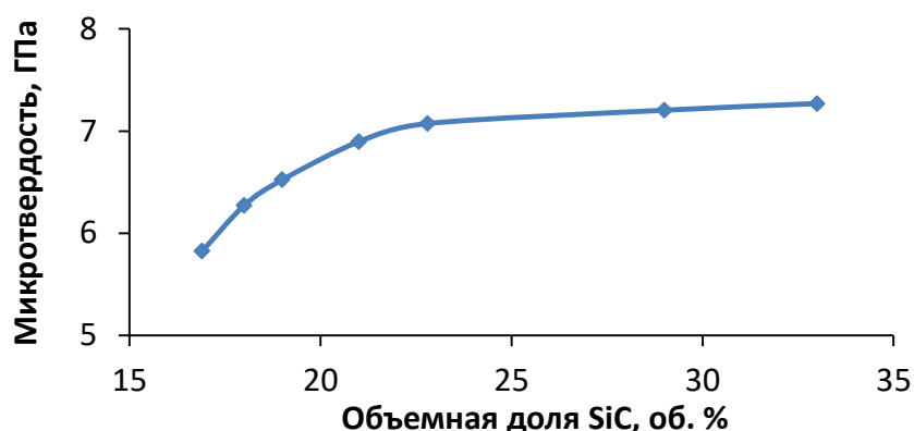
Рисунок 5.20 – Влияние объемной доли субмикронного карбида кремния на микротвердость композиционного покрытия Ni-SiC
