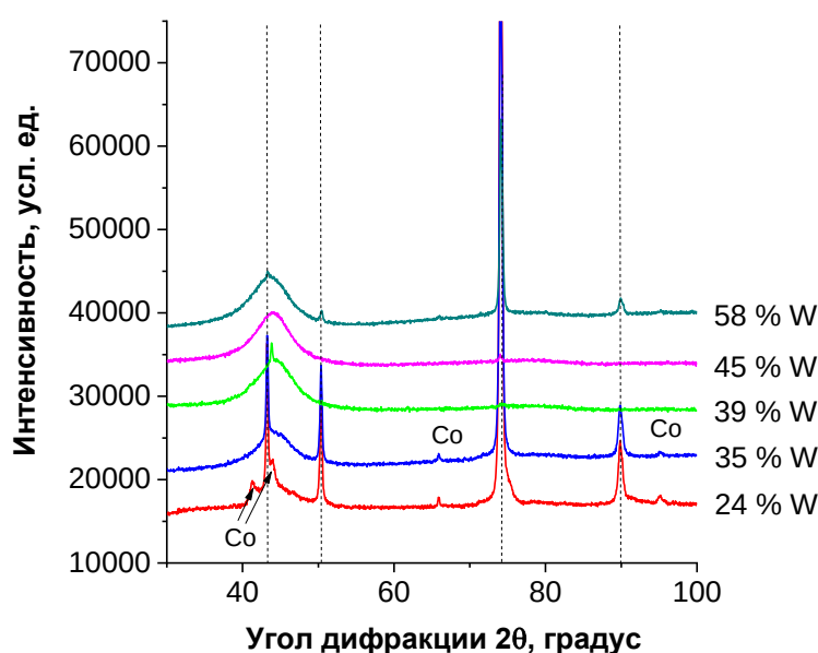
Рисунок 3.42 – Рентгеновские дифрактограммы покрытий Co-W с различным содержанием вольфрама (в мас. %). Штрихпунктирной линией обозначены рефлексы от медной основы образцов
