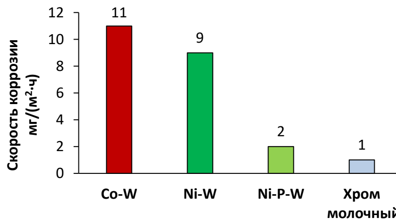
Рисунок 7.3 – Средняя скорость коррозии (за 300 ч) при экспозиции разработанных кристаллизационных покрытий в 3,5 %-ном растворе NaCl
