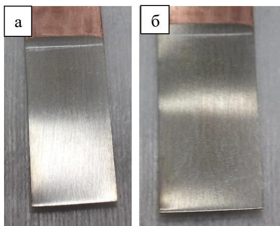
Рисунок 3.18 – Медные образцы с покрытием Ni-44 мас. % W толщиной 10 мкм в 70 % \text{HNO}_3 : а) до экспозиции; б) после экспозиции 300 с
