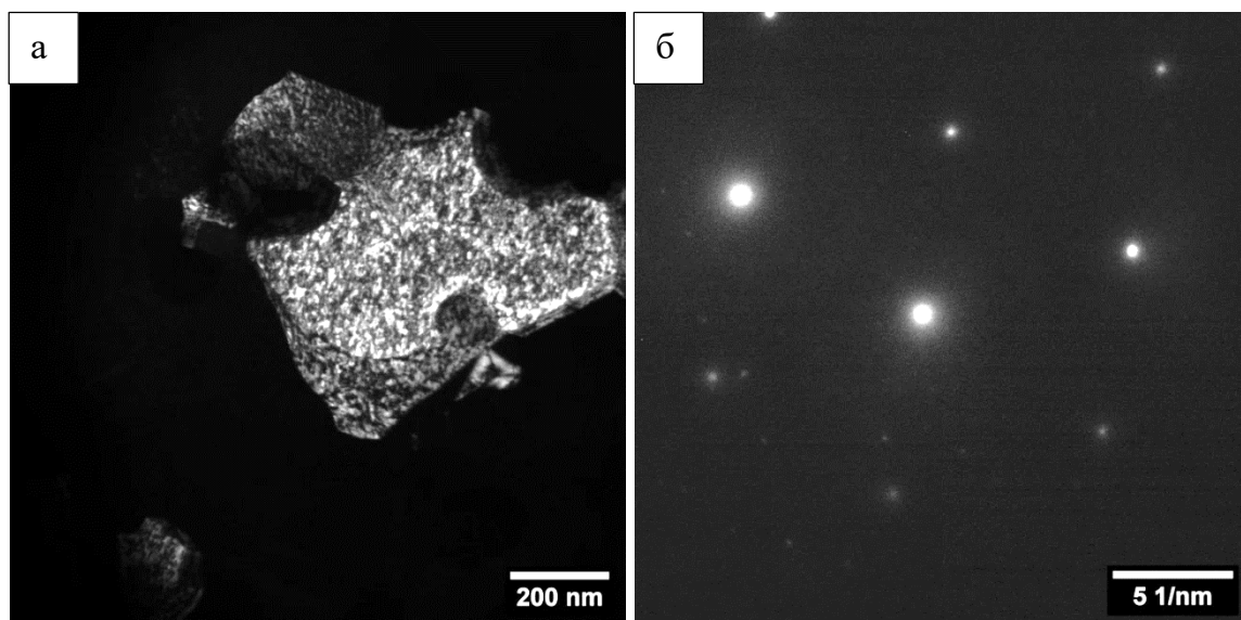
Рисунок 3.33 – Микроструктура матрицы покрытия Ni-44 мас. % W, термообработанного при 750 °С в течение 5 ч: а) темнопольное изображение; б) электронограмма от твердого раствора
