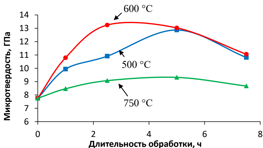
Рисунок 3.24 – Влияние продолжительности термообработки на микротвердость покрытия Ni-44 мас. % W при различных температурах
