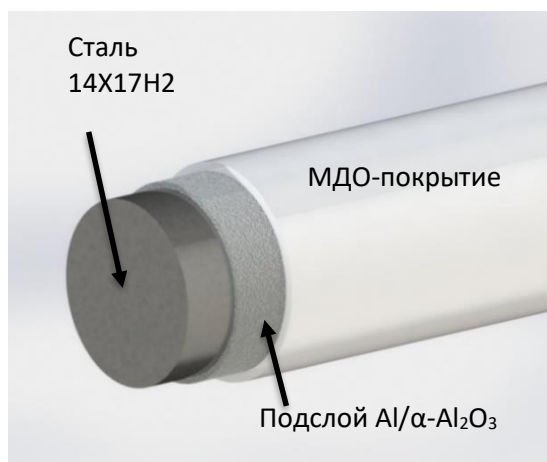
Рисунок 6.13 – Схема конверсионного композиционного покрытия на стальном образце
