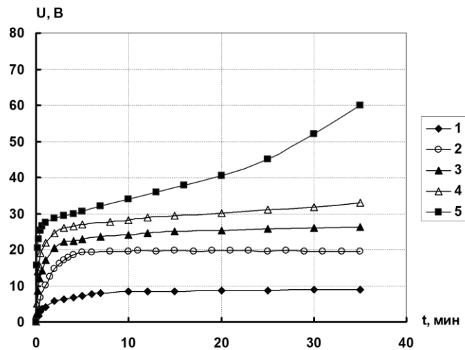
Рисунок 6.7 – Изменение во времени напряжения на ванне анодирования силумина АК7ч в перемешиваемом электролите 3 при температуре электролита 18 °С и различной плотности тока: 1 – 0,5 А/дм 2 ; 2 – 1,0 А/дм 2 ; 3 – 2,0 А/дм 2 ; 4 – 3,0 А/дм 2 ; 5 – 5,0 А/дм 2 .
