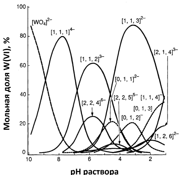
Рисунок 3.1 – Распределение комплексов [(\text{WO}_4^{2-})_x(\text{Cit}^{3-})_y(\text{H}^+)_z]^{n-} в зависимости от pH, где x , y , z – стехиометрические коэффициенты для компонентов комплексного соединения, n – заряд комплексного иона [324]
