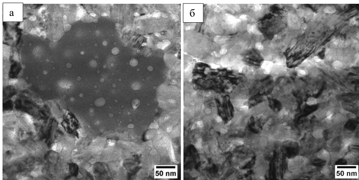
Рисунок 3.54 – Поры в покрытиях Co-W после термообработки при 750 °С в течение 5 ч: а) в частице (\text{Fe}, \text{Co})_6\text{W}_6\text{C} ; б) в интерметаллиде \text{Co}_3\text{W}
