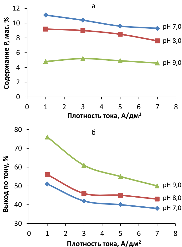
Рисунок 4.5 – Влияние pH цитратного электролита на содержание фосфора в покрытии Ni-P (а) и его выход по току (б) при концентрации гипохлорита натрия 0,05 моль/л
