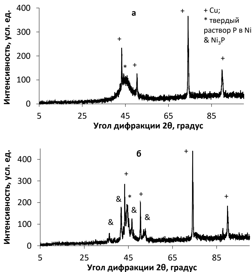
Рисунок 4.9 – Рентгеновские дифрактограммы покрытия Ni-10,2 % P, осажденного из электролита с 0,10 моль/л \text{NaH}_2\text{PO}_2 при плотности тока 4 А/дм 2 : а) в исходном состоянии; б) после термообработки при 350 °С, 1 ч
