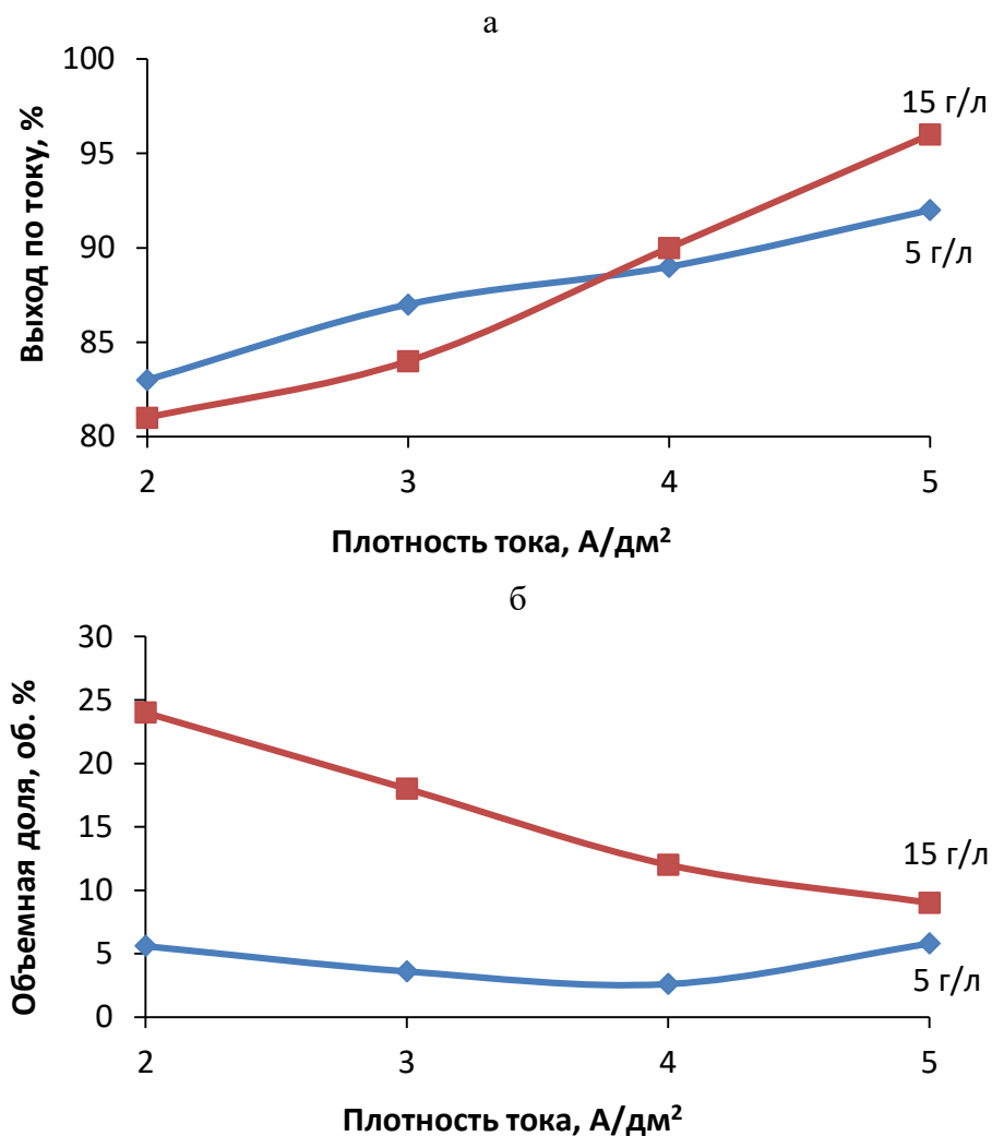
Рисунок 5.5 – Влияние плотности тока на выход по току композиционного покрытия (а) и содержание карбида кремния (б) в условиях вибрационного перемешивания при различной концентрации SiC.
