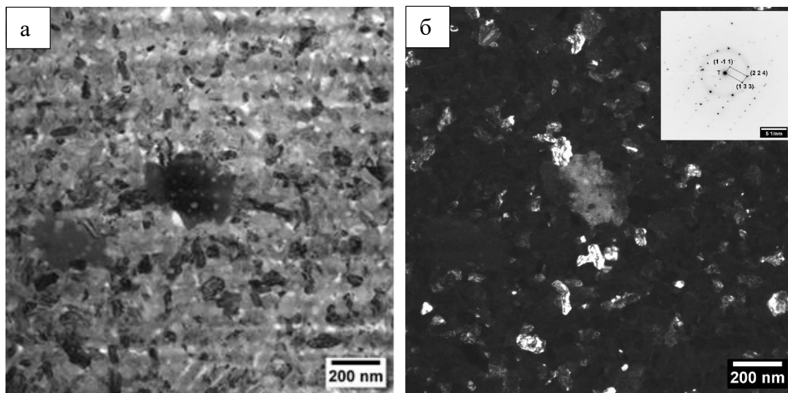
Рисунок 3.53 – Частица (\text{Fe}, \text{Co})_6\text{W}_6\text{C} в нанокристаллической матрице \text{Co}_3\text{W} : а) светлопольное изображение; б) темнопольное изображение в рефлексе (3 3 3)
