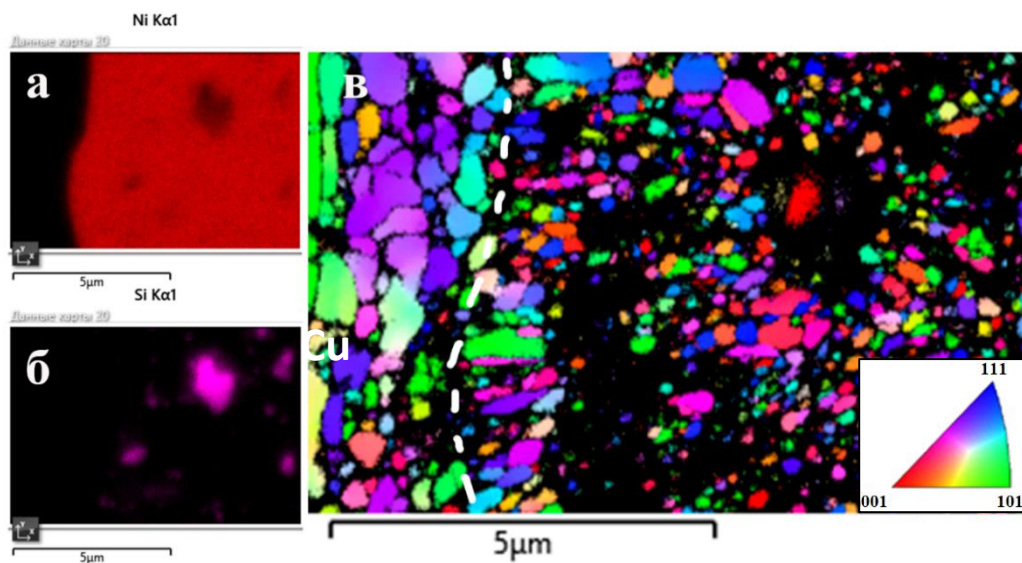
Рисунок 5.28 – Структура матрицы покрытия Ni-SiC на поперечном шлифе вблизи границы раздела с медной основой: а) карта распределения Ni; б) карта распределения Si; в) визуализация микроструктуры матрицы с помощью метода ДОРЭ
