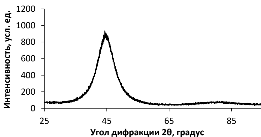
Рисунок 4.14 – Рентгеновская дифрактограмма покрытия Ni-P-W до термообработки
