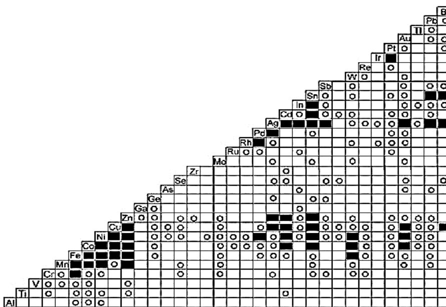
Рисунок 1.1 – Пары металл – металл, которые возможно осадить электрохимическим способом: ○ – получены лабораторные образцы; ■ – сплавы, представляющие технический интерес либо широко используемые [18]
